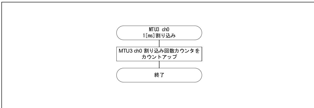
図 3-15 マルチファンクションタイマパルスユニット 3 (チャンネル 0) 1 [ms]割り込み処理フローチャート
