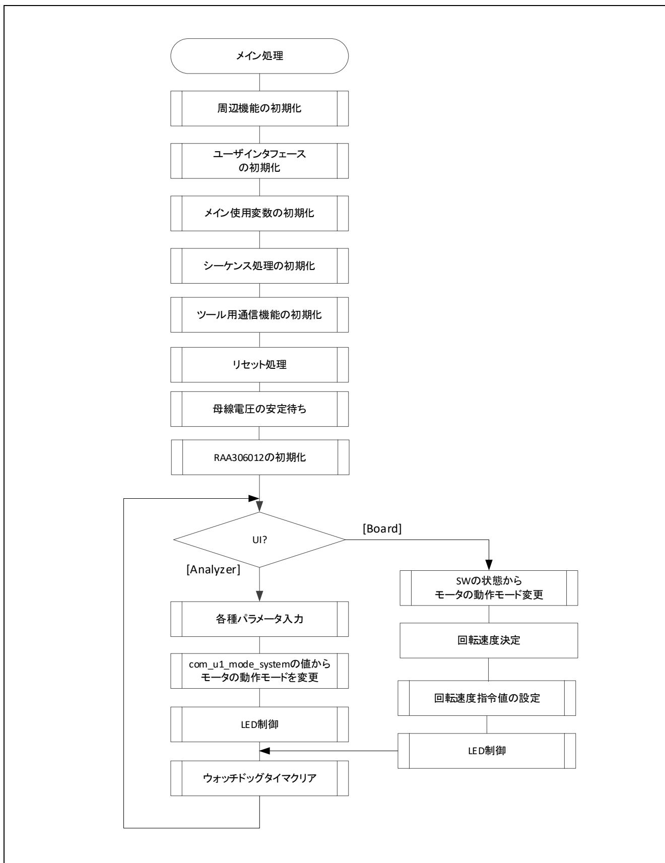
図 3-7 メイン処理フローチャート
