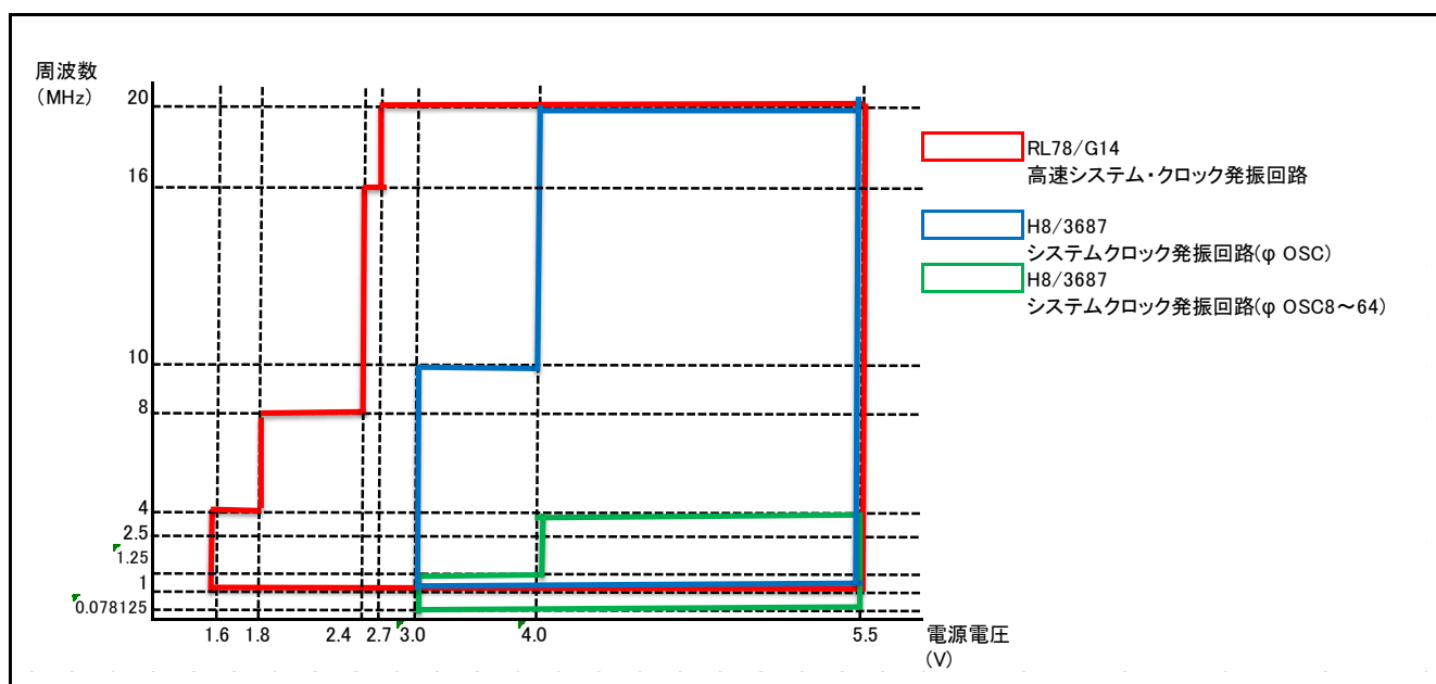
図1.1 システムクロック発振回路の動作周波数比較
