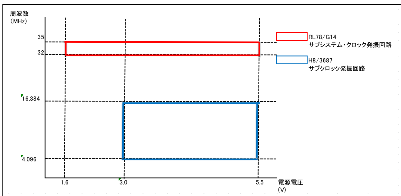
図1.3 XCIN クロック発振回路の動作周波数比較
