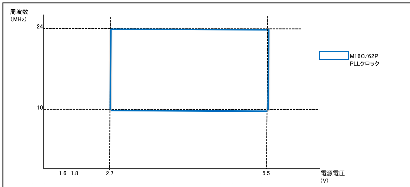
図1.5 PLL クロックの動作周波数比較
