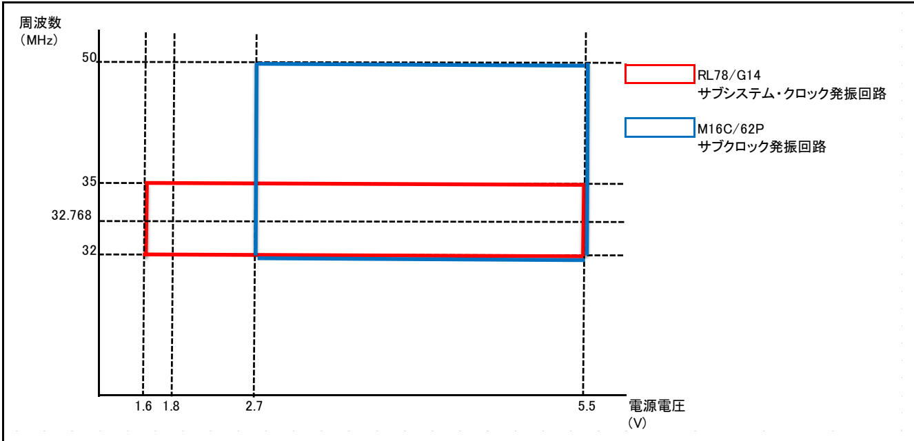
図1.3 サブクロック発振回路の動作周波数比較
