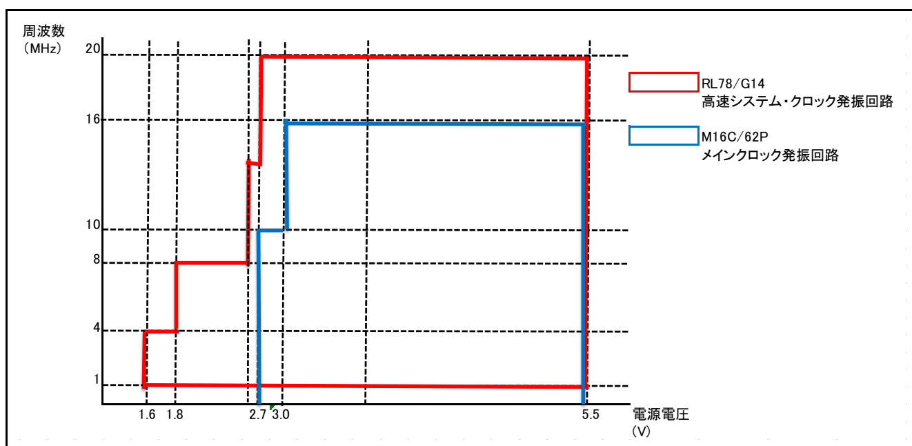
図1.1 メインクロック発振回路の動作周波数比較
