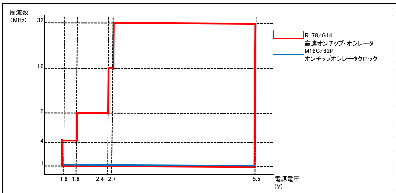
図1.2 高速オンチップオシレータの動作周波数比較
