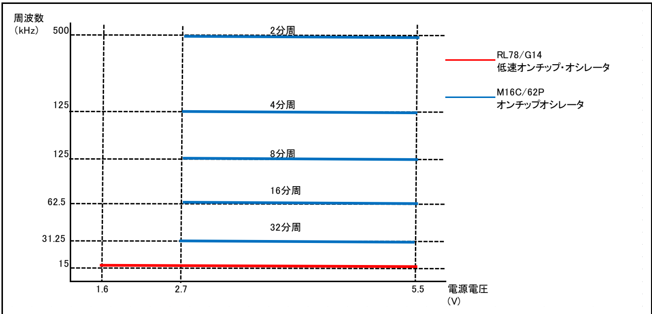
図1.4 低速オンチップオシレータの動作周波数比較
