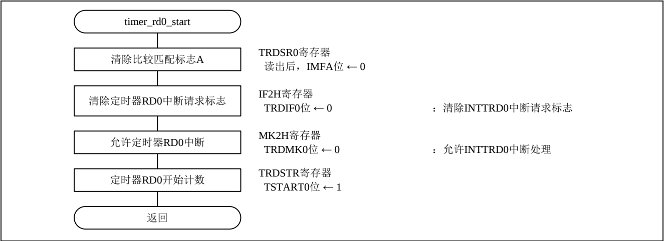
图 4.9 定时器 RD 计数开始设置
