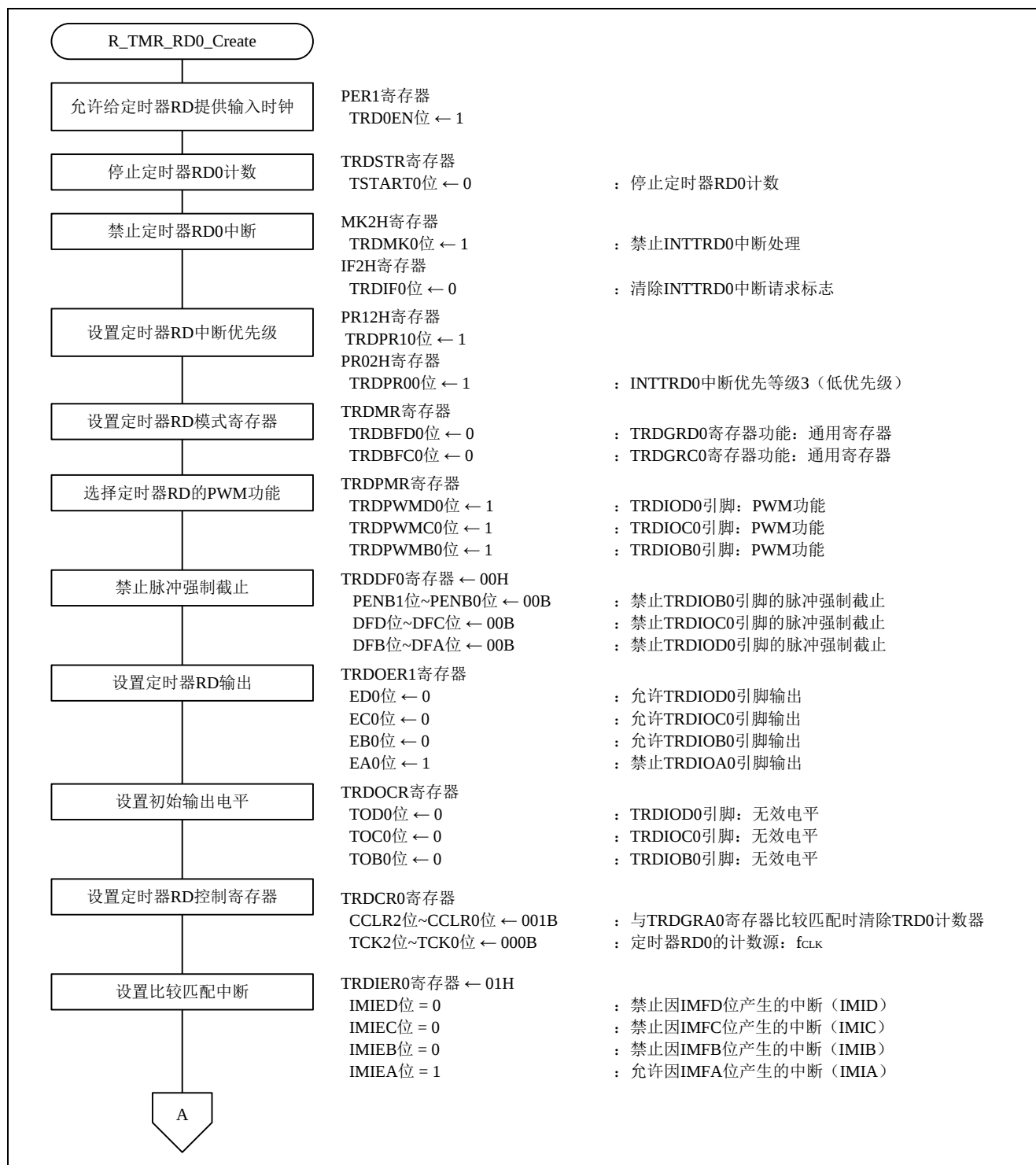
图 4.6 定时器 RD 初始化设置（1/2）
