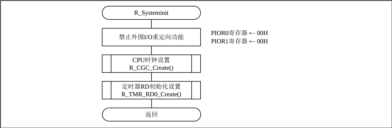
图 4.4 系统函数
