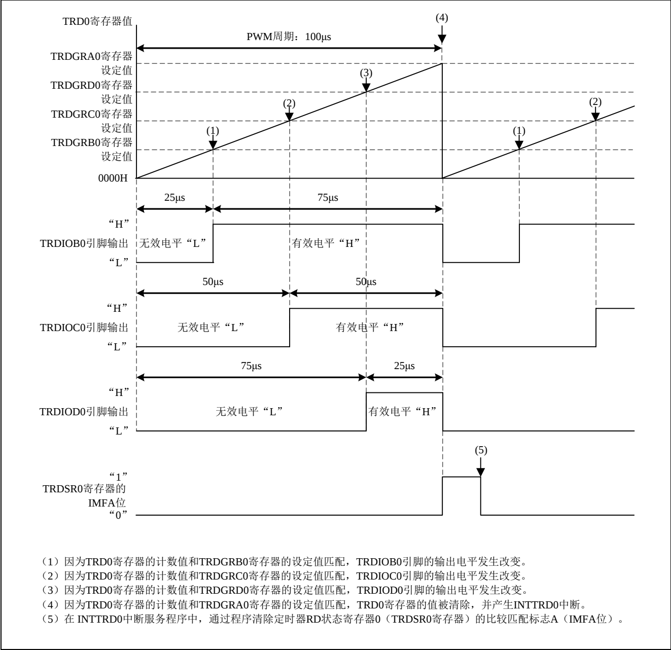
图 4.1 PWM 输出波形
