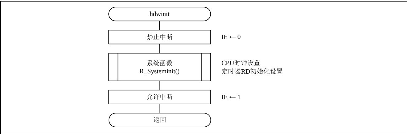
图 4.3 初始化设置
