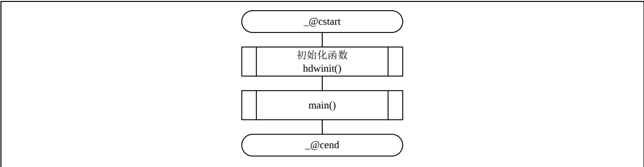
图 4.2 整体流程图
