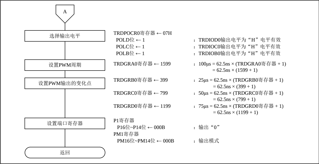
图 4.7 定时器 RD 初始化设置 (2/2)
