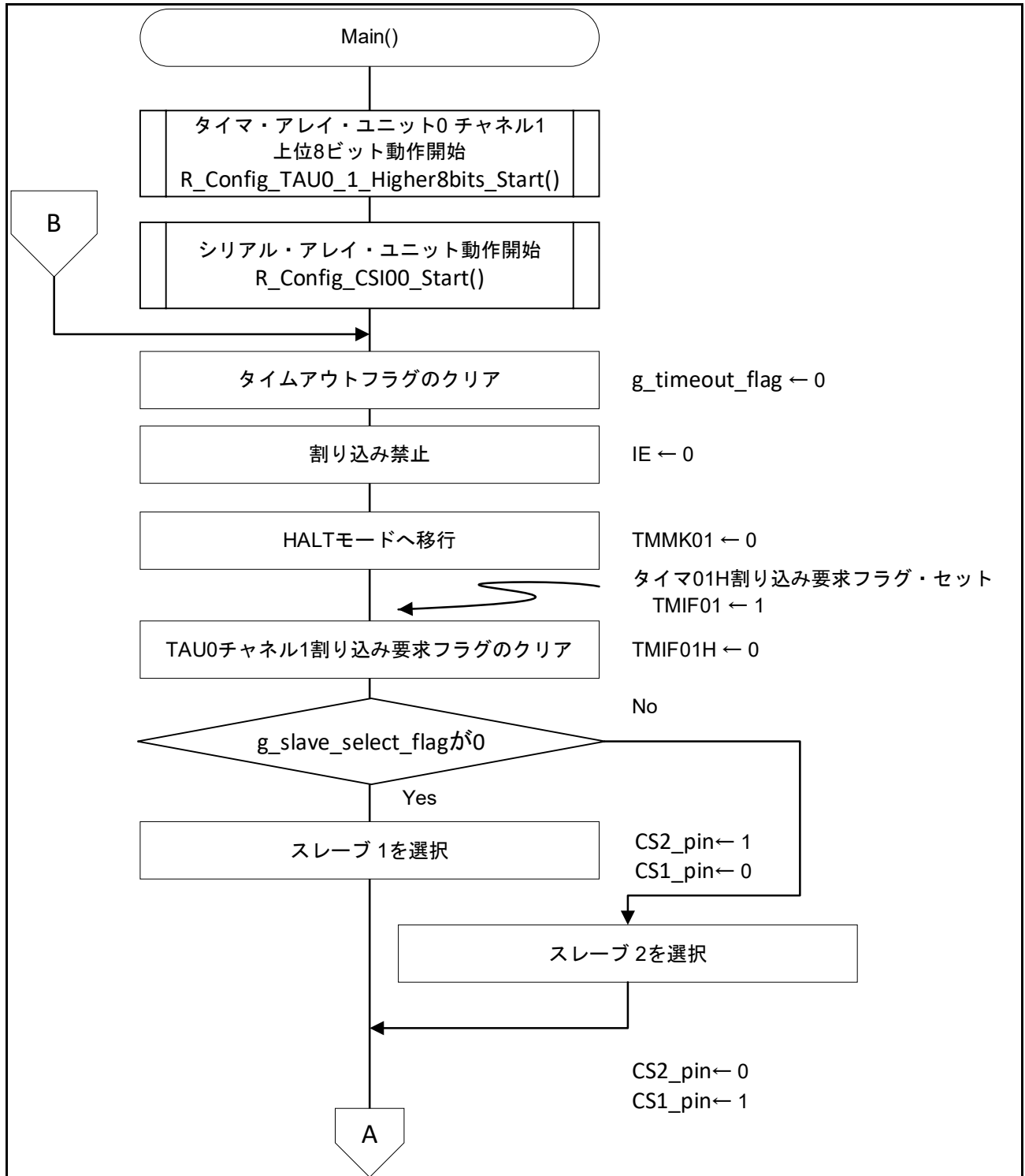
図 5-1 メイン処理 1/2
