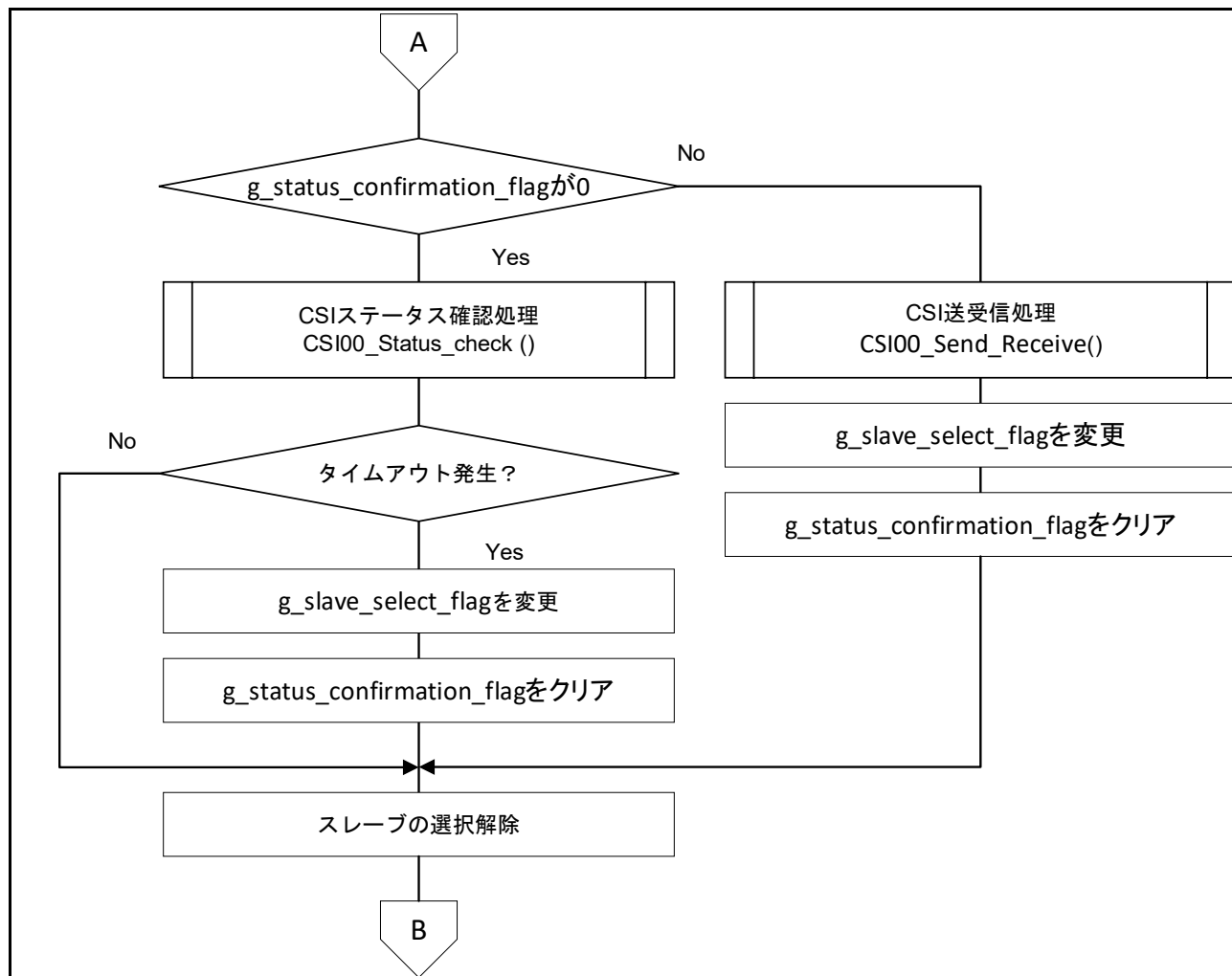
図 5-2 メイン処理 2/2
