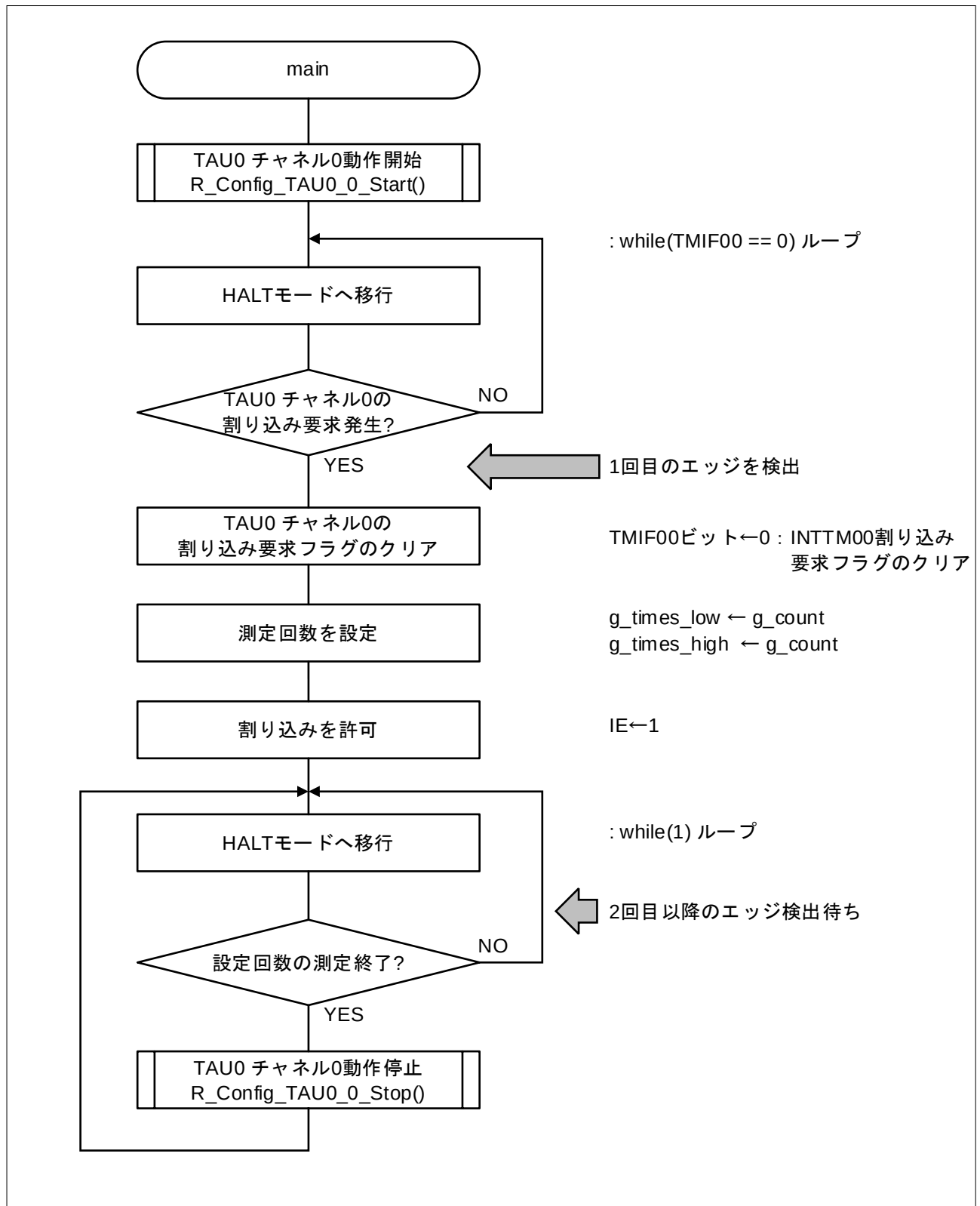
図 4-1 メイン処理
