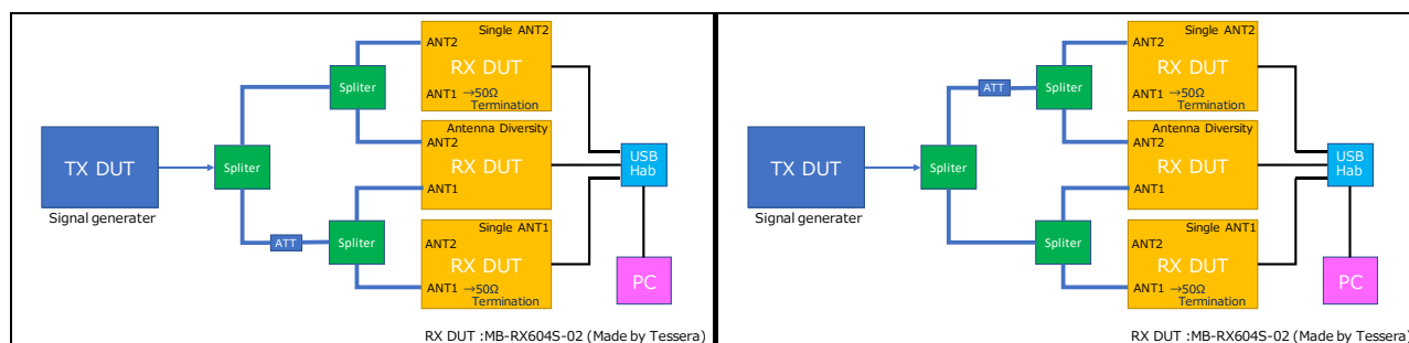
Figure 2. ATT on ANT1 side
