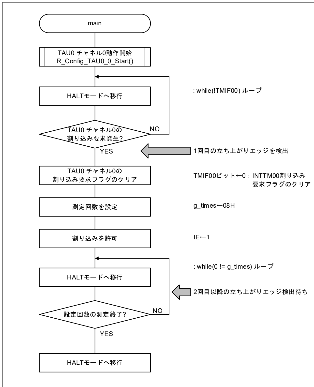
図 4-1 メイン処理
