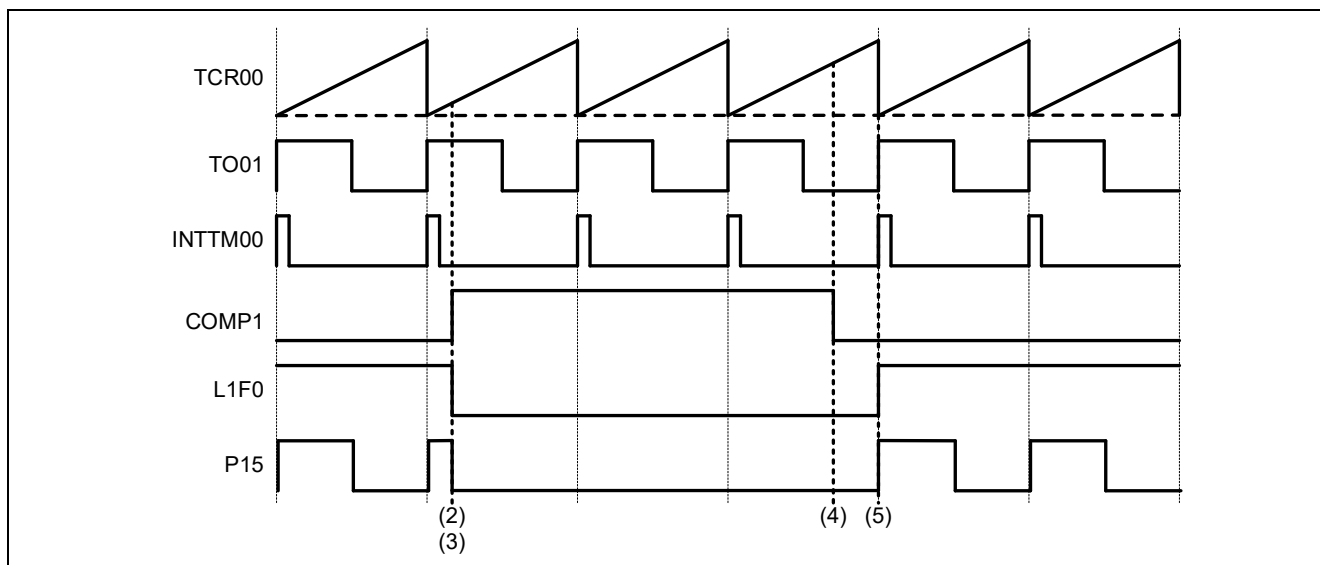
図 5-4 タイミングチャート
