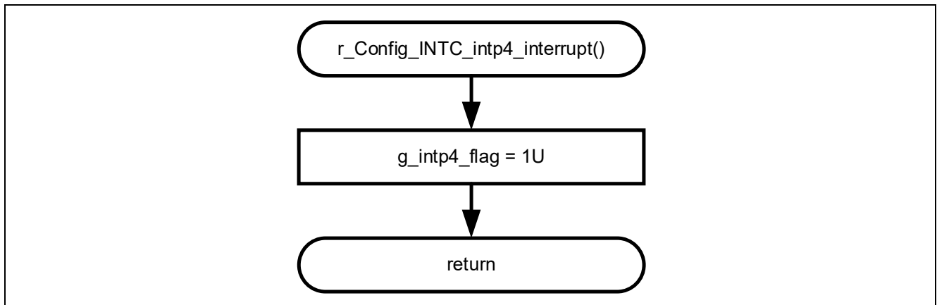
図 4-4 INTP4 割り込み処理
