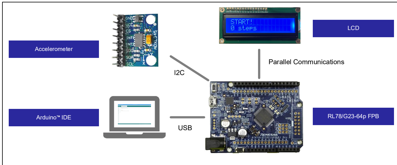
図 1-2 開発時のシステム構成図
