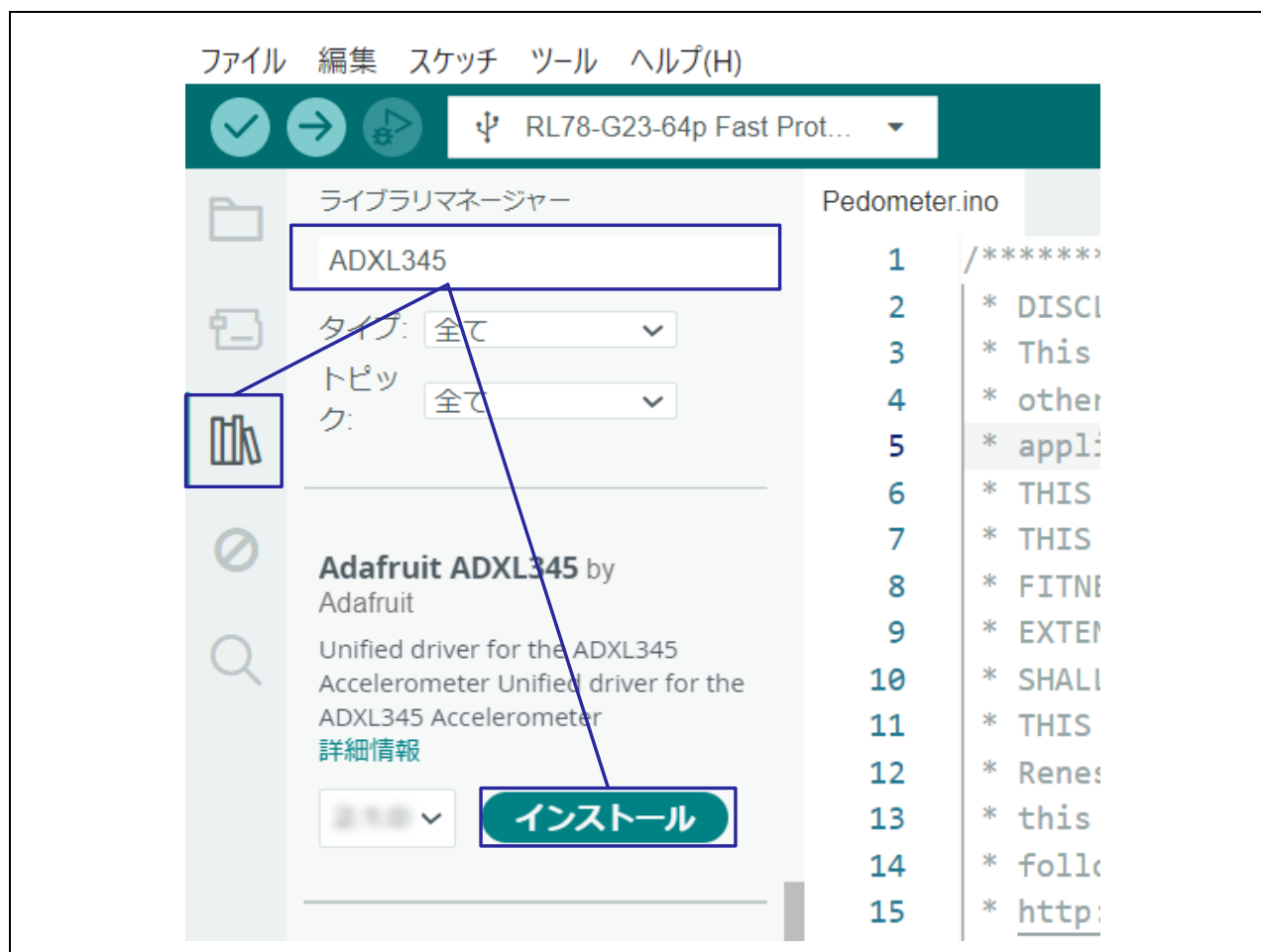
図 4-5 Adafruit_ADXL345 のインストール
