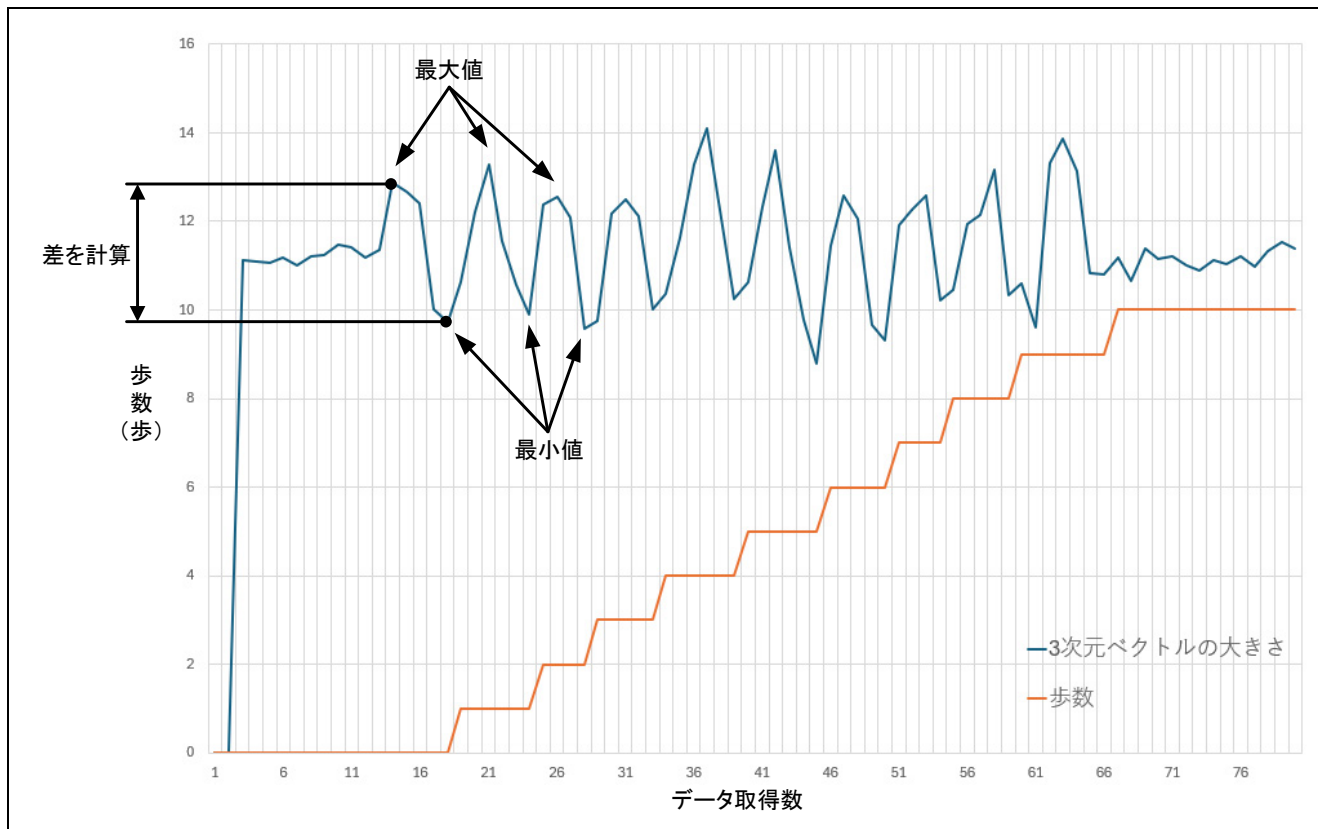
図 4-4 歩数のカウント
