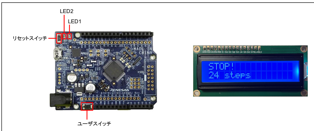
図 4-13 LED1 とスイッチの位置と歩数計測終了時の LCD モジュールの表示
