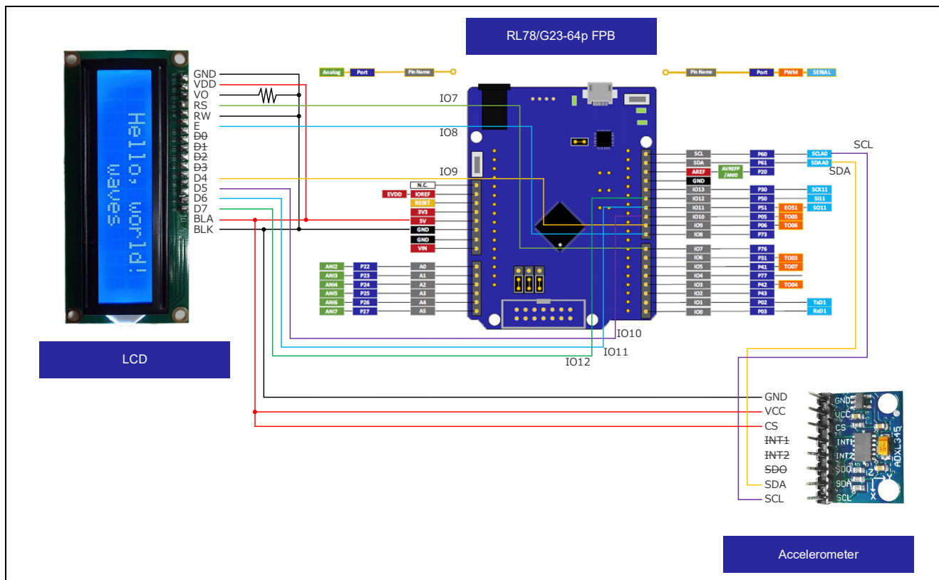
図 3-1 評価ボード、加速度センサ、LCD モジュールの接続
