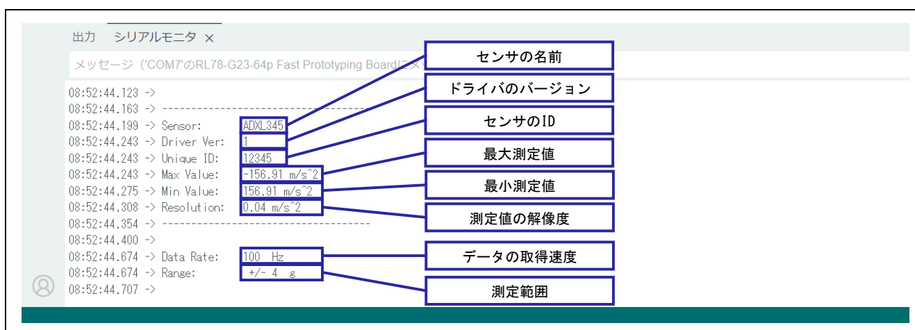
図 4-2 開発時にシリアルモニタに表示される内容
