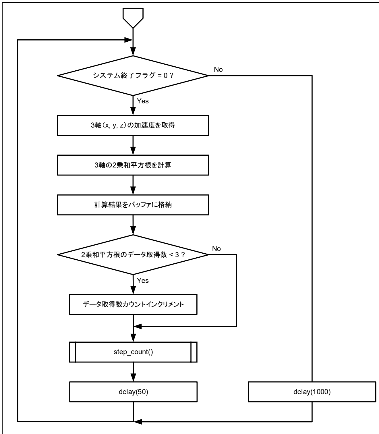
図 4-15 メイン処理フローチャート(2/2)
