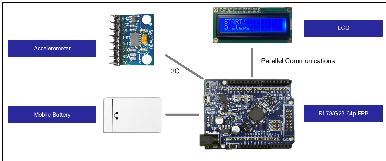
図 1-3 歩数計測時のシステム構成図
