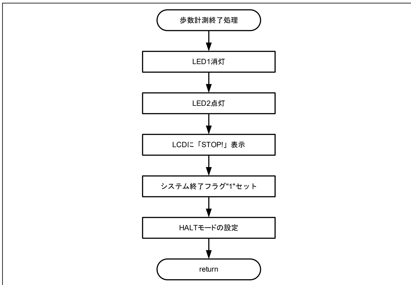
図 4-17 stop_system 関数のフローチャート
