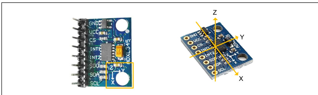
図 1-4 加速度センサと各軸の測定方向
