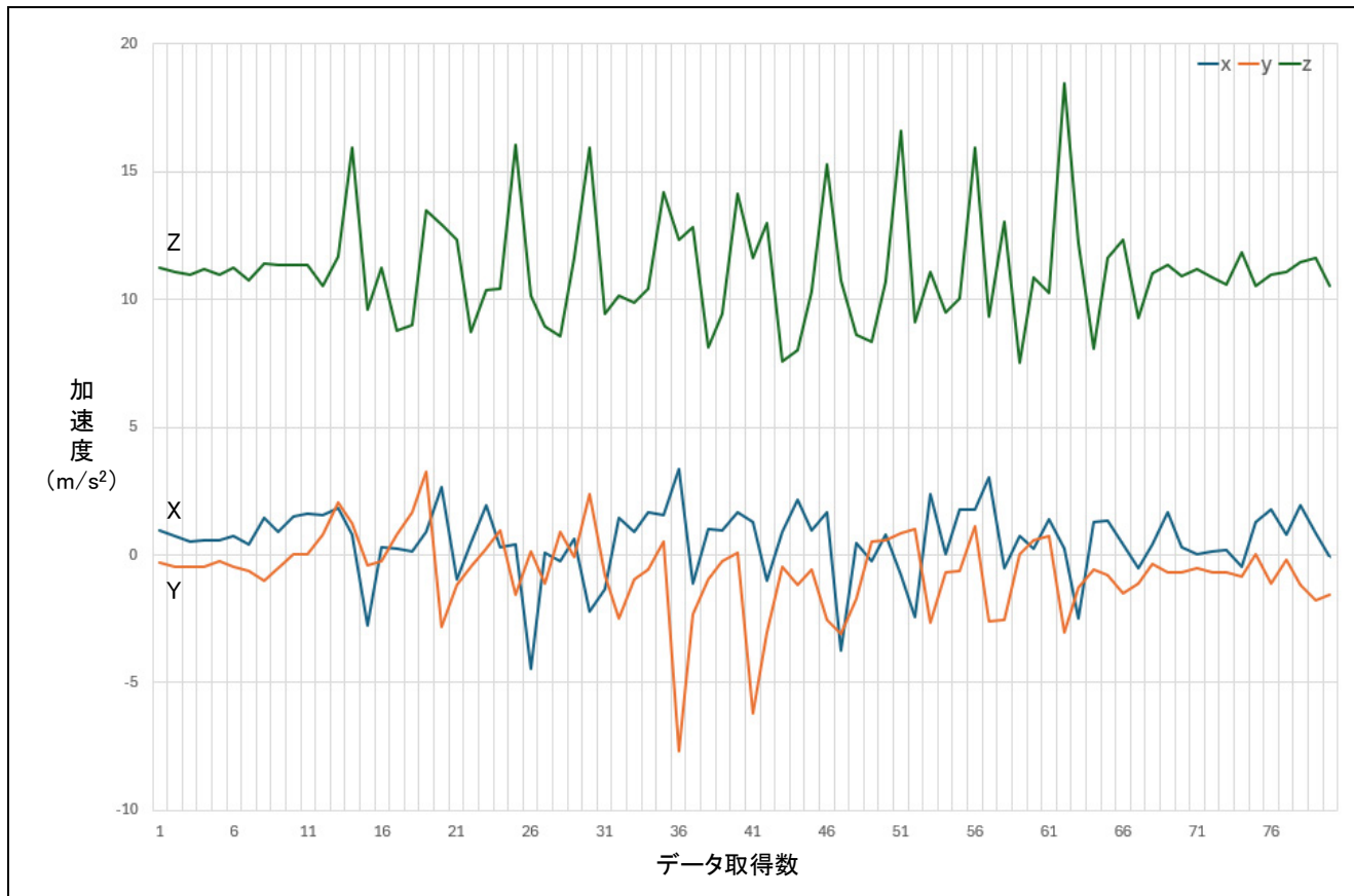
図 4-3 歩行時の 3 軸の加速度の変化
