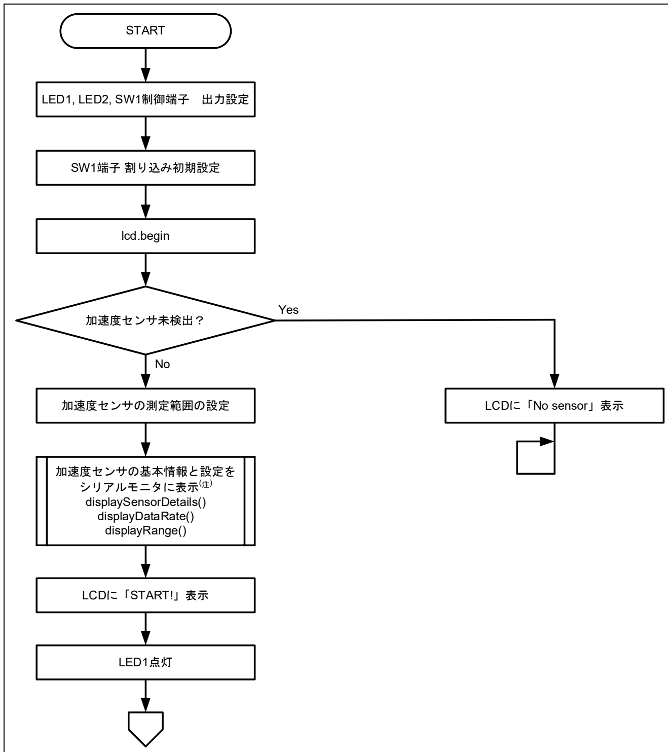
図 4-14 メイン処理フローチャート(1/2)
