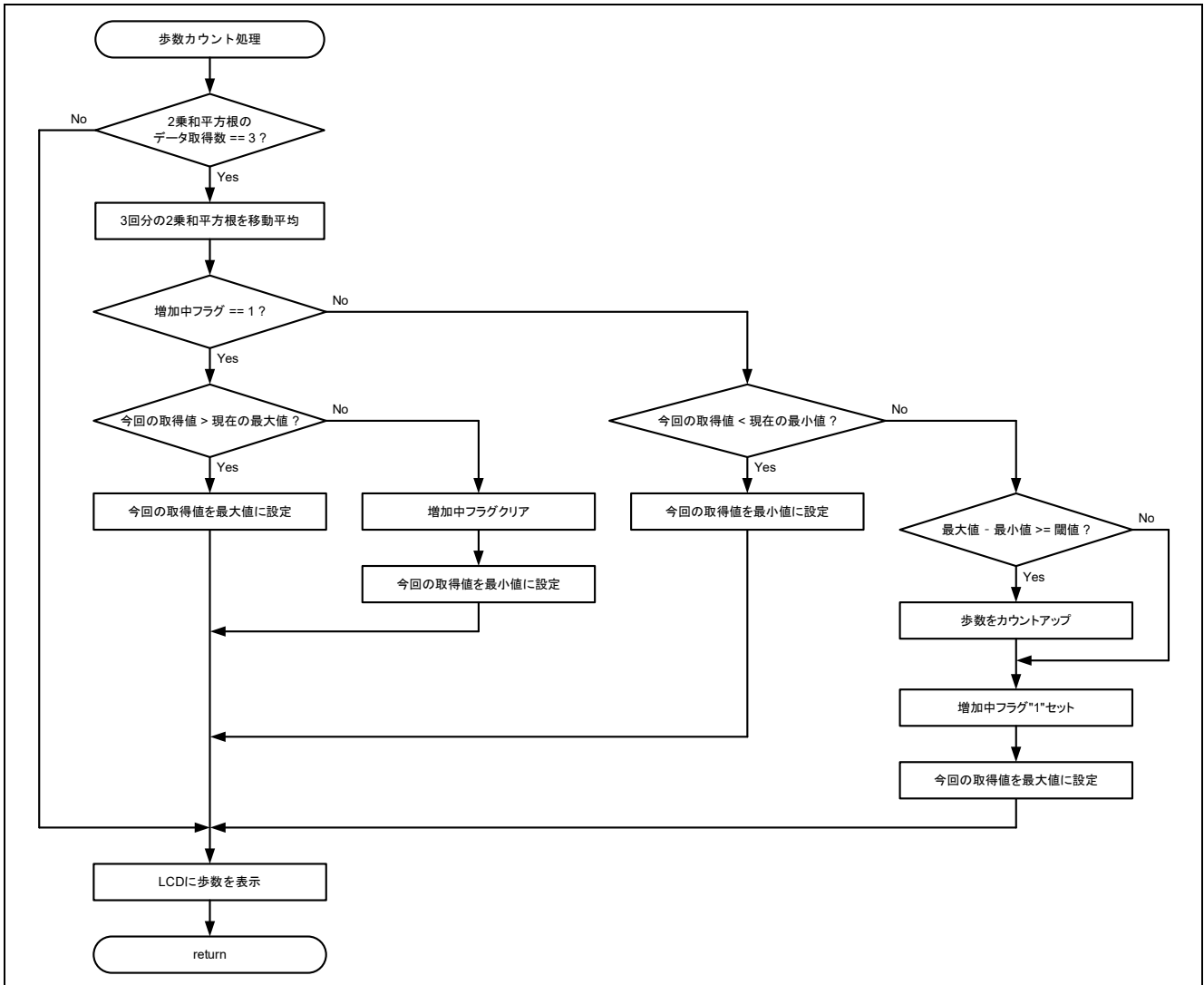
図 4-16 step_count 関数のフローチャート
