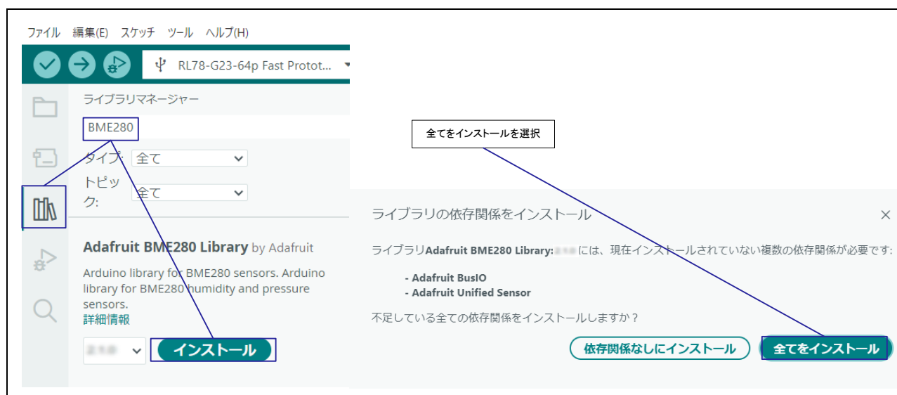
図 4-2 Adafruit BME280 Library のインストール
