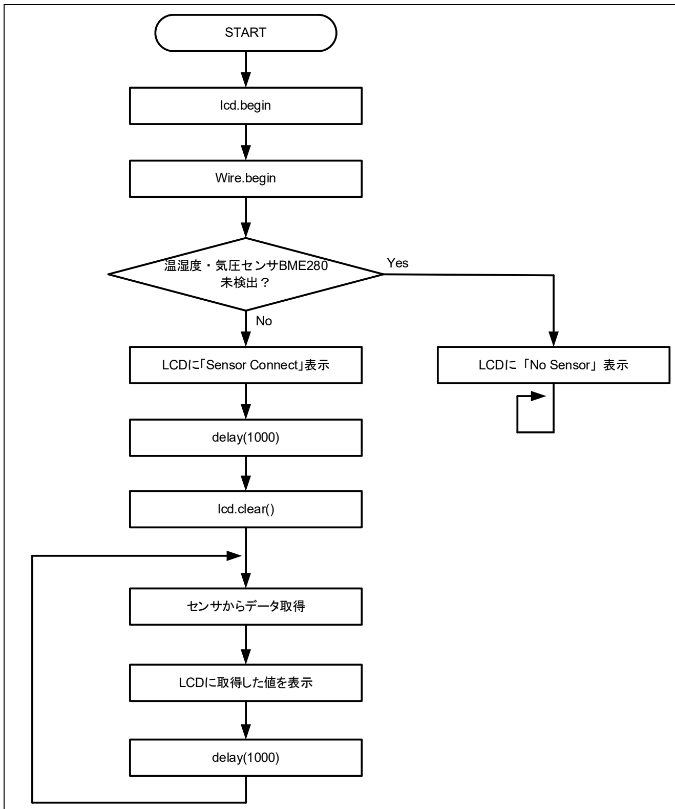
図 4-11 メイン処理フローチャート
