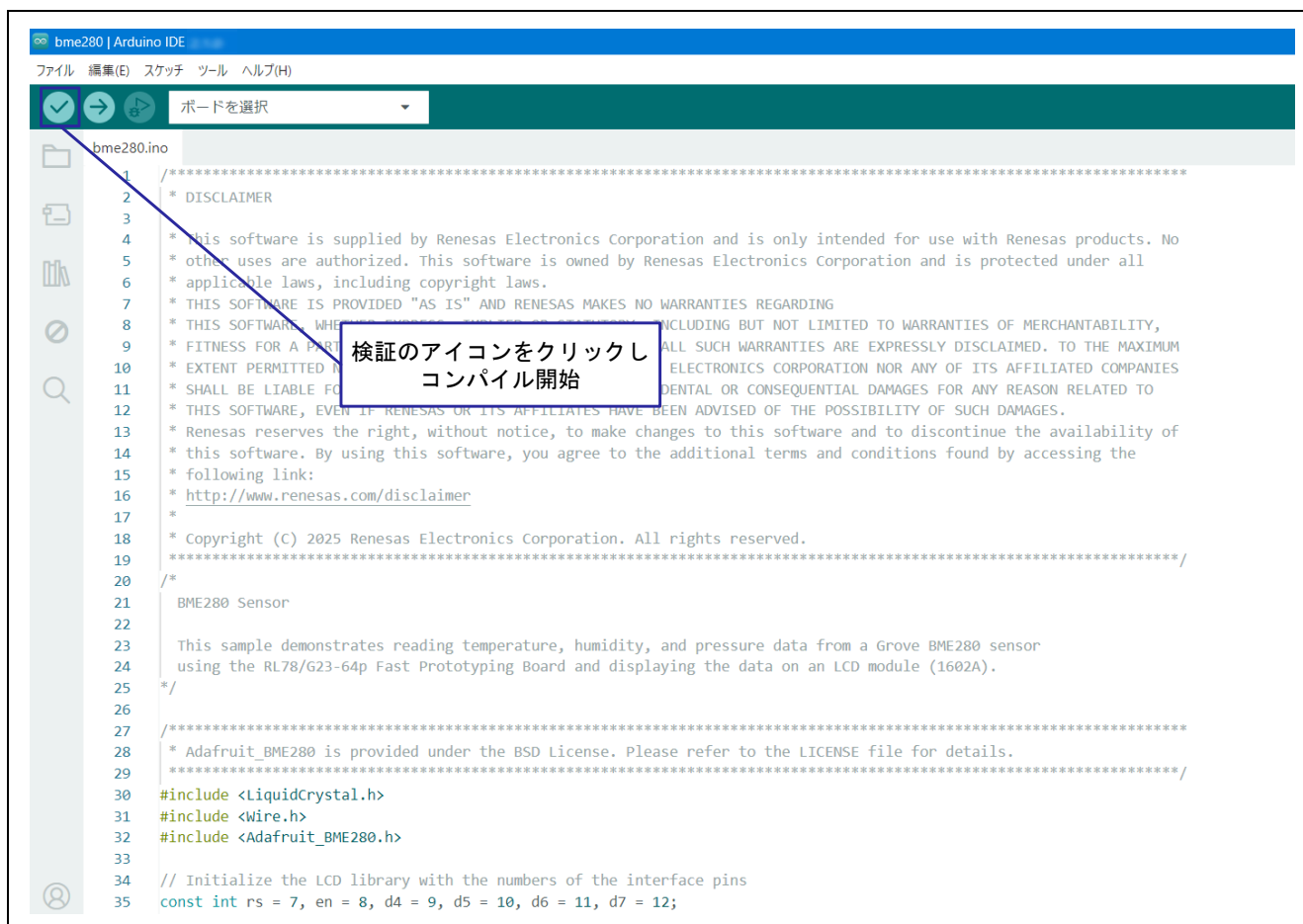
図 4-6 スケッチのコンパイル
