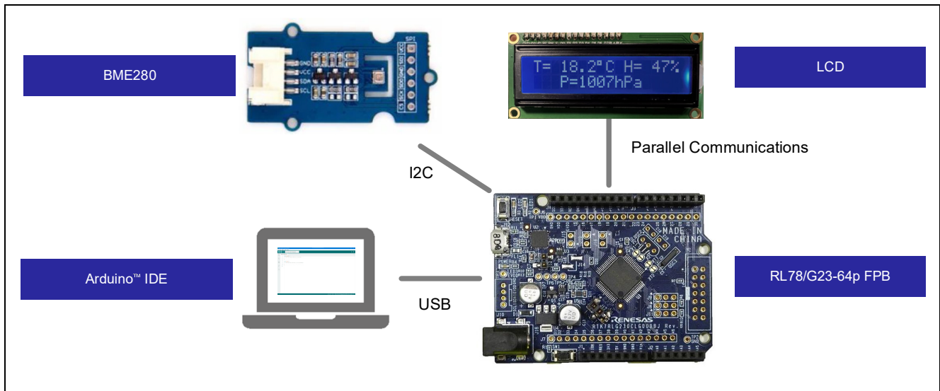
図 1-2 システム構成図
