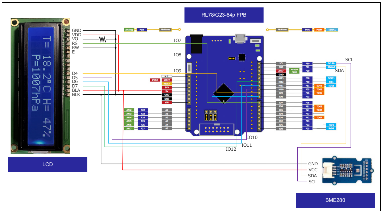
図 3-1 評価ボード、BME280、LCD モジュールの接続
