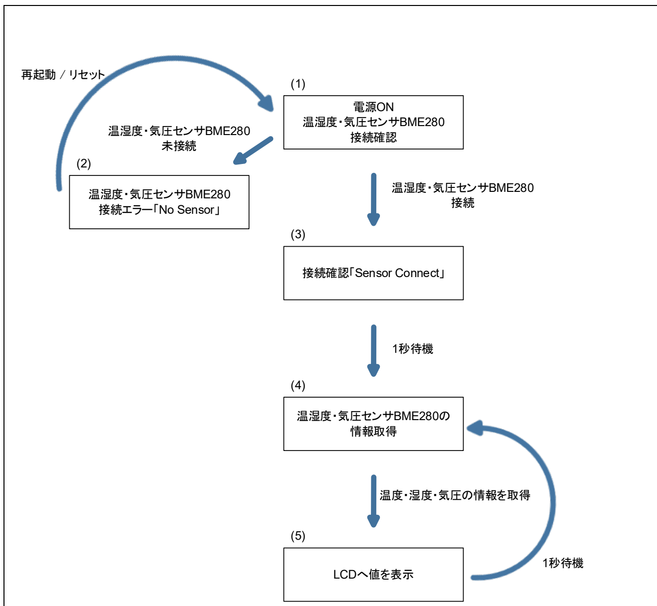
図 1-5 動作概要
