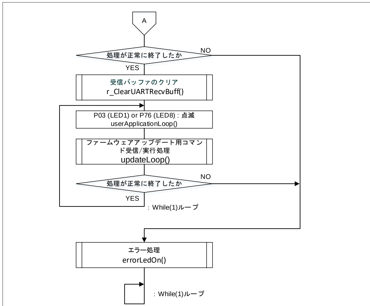
図 4-2 メイン処理 (2/2)
