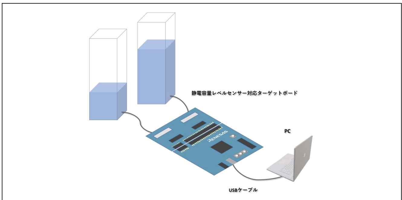
図 2.1 機器接続図
