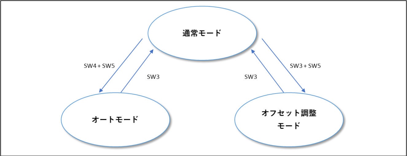
図 6.1 モード遷移
