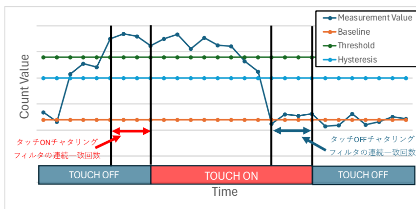
図 4 チャタリング防止処理
