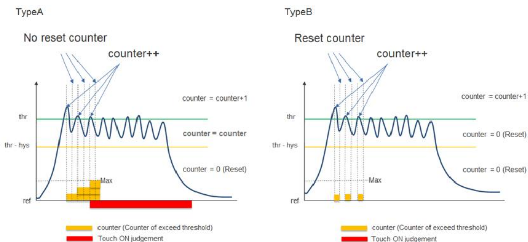
図 5 チャタリング防止タイプ
