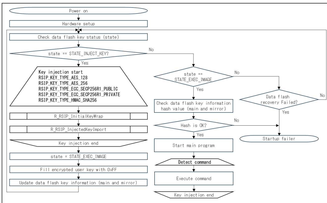
図 6-2 鍵注入と暗号の使用方法のデモプロジェクトの動作フロー
