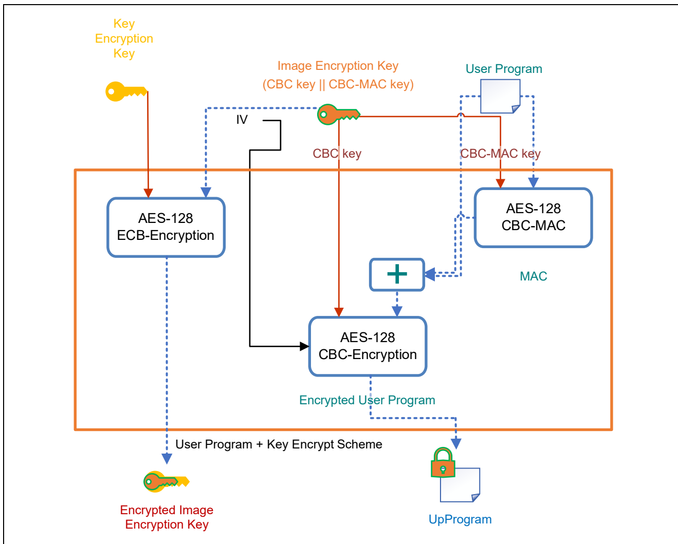
図 3-10 ファームウェアと Image Encryption Key の暗号化方法
