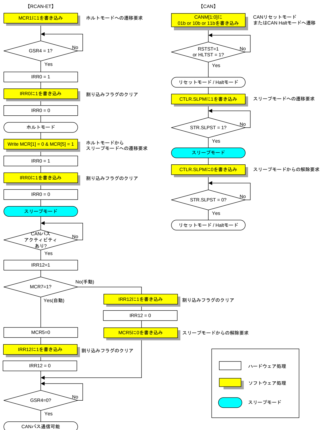
図 1 SH7137 (RCAN-ET) と RX65N (CAN) のスリープモードへの設定手順
