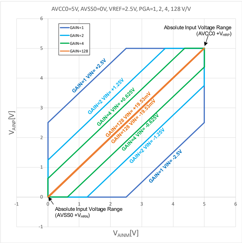
図 2-1 DSAD への入力電圧範囲 (5V 入力端子の場合)
