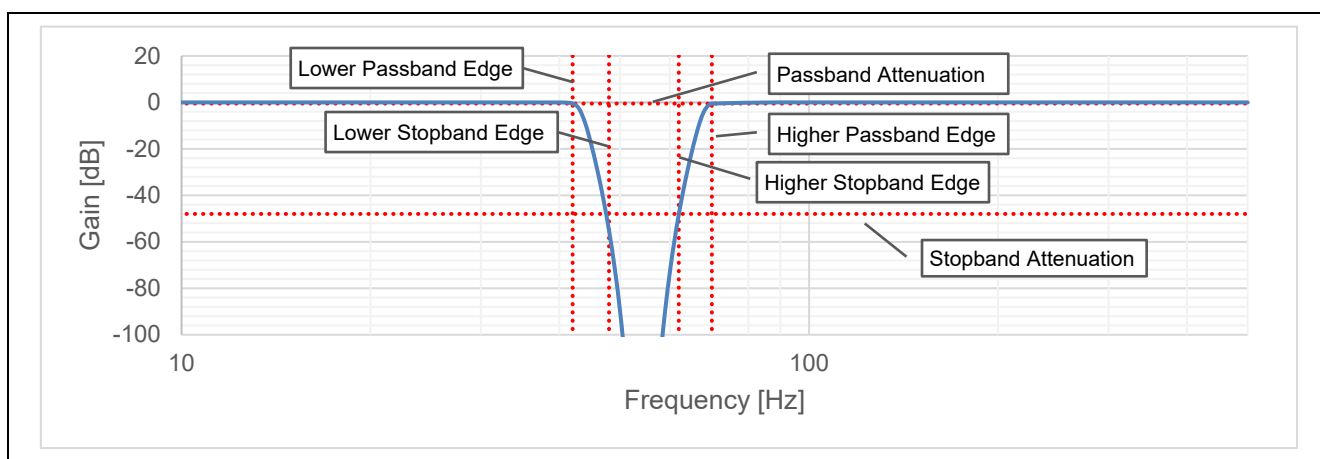
図 1-7 バンドエリミネータフィルタ周波数特性
