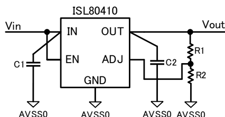
図 2-8 LDO の電源デカップリング例
