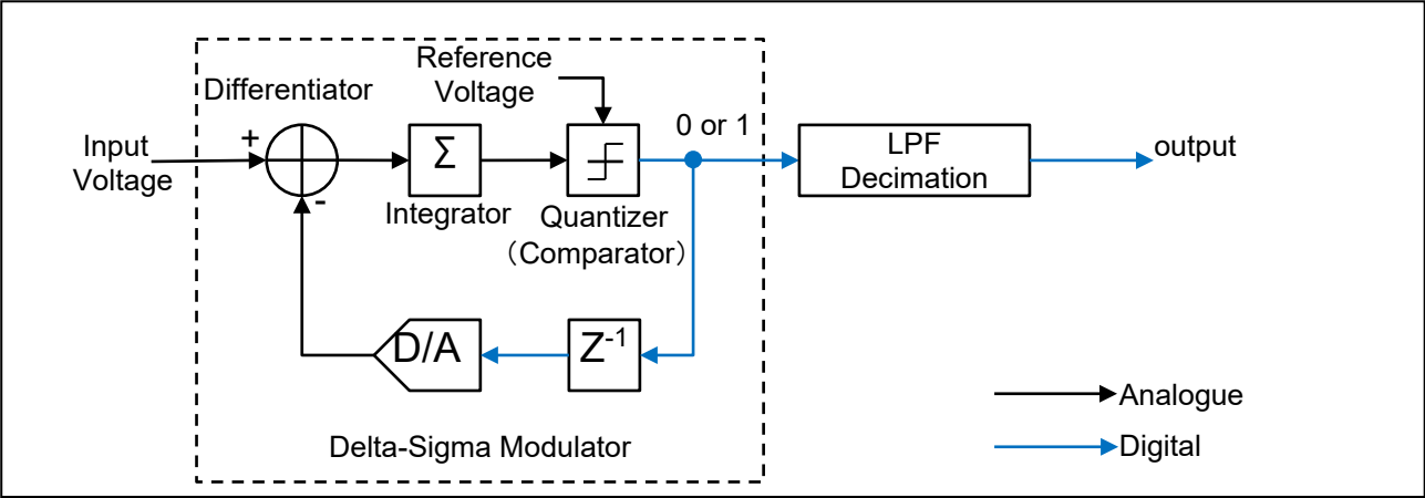
図 1-1 \Delta - \Sigma A/D コンバータ原理図
