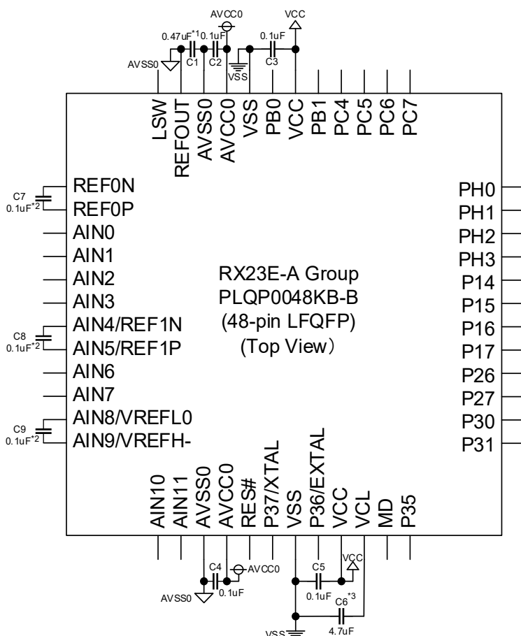
図 2-8 LDO の電源デカップリング例
