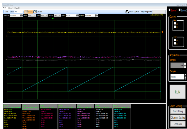
図 5-1 TAD2141 を使用した速度制御波形
