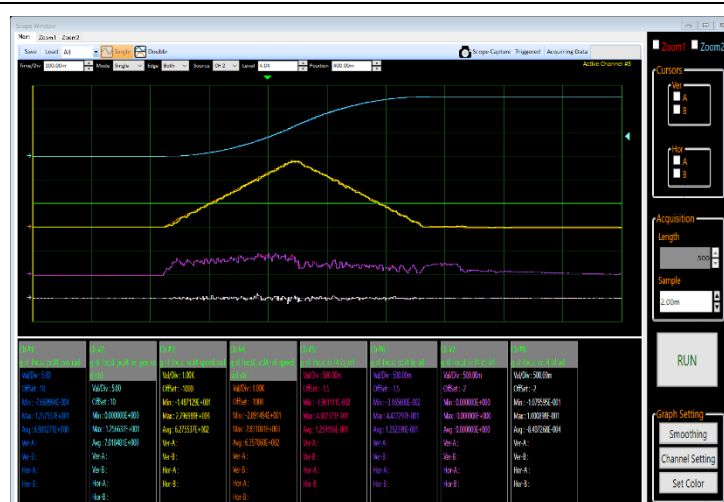
図 5-2 TAD2141 を使用した位置制御波形
