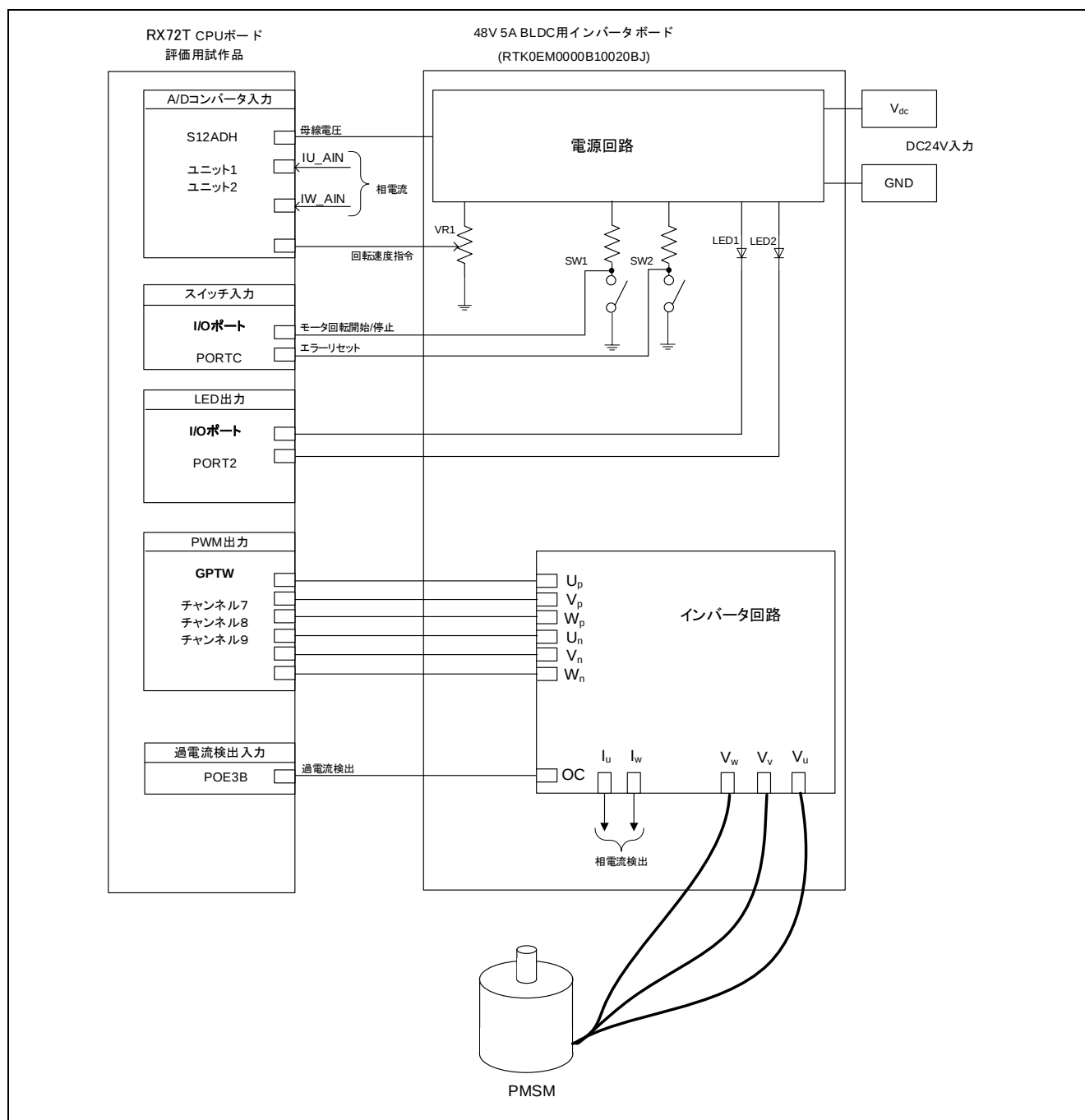
図 2-6 モータ 4 向けハードウェア接続構成図
