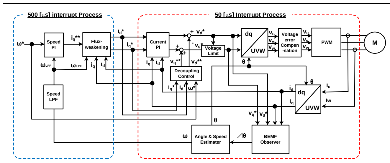
図 3-6 センサレスベクトル制御概略ブロック図（センサレス制御時）
