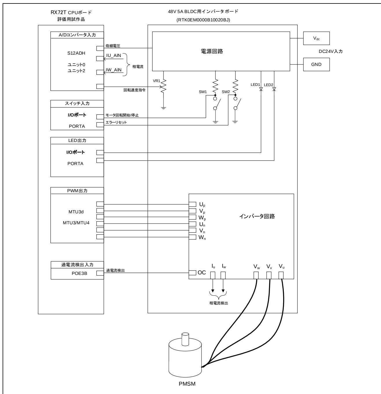
図 2-3 モータ 1 向けハードウェア接続構成図
