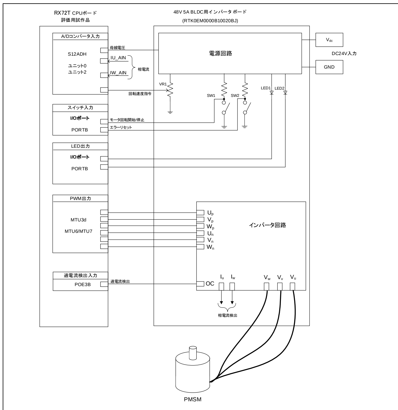
図 2-4 モータ 2 向けハードウェア接続構成図
