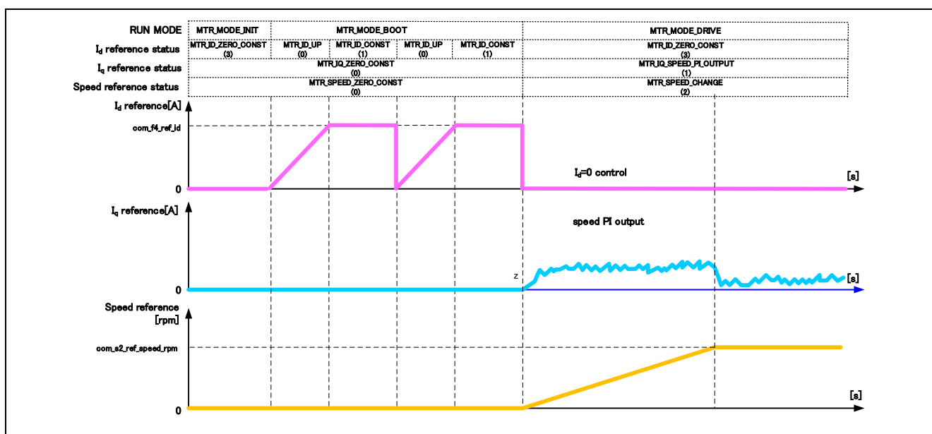
図 3-8 エンコーダ利用ベクトル制御ソフトウェアの始動制御内容（速度制御時）
