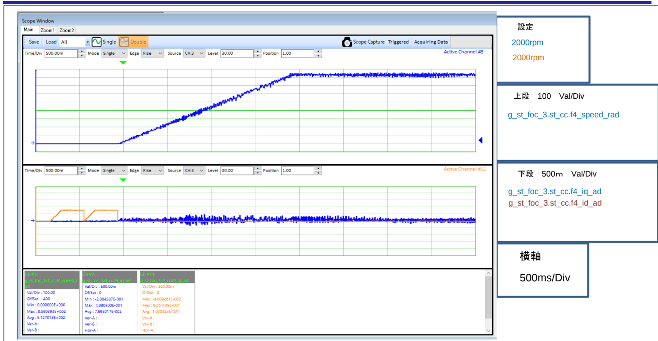
図 5-3 起動時駆動波形（3/3）（モータ 3）
