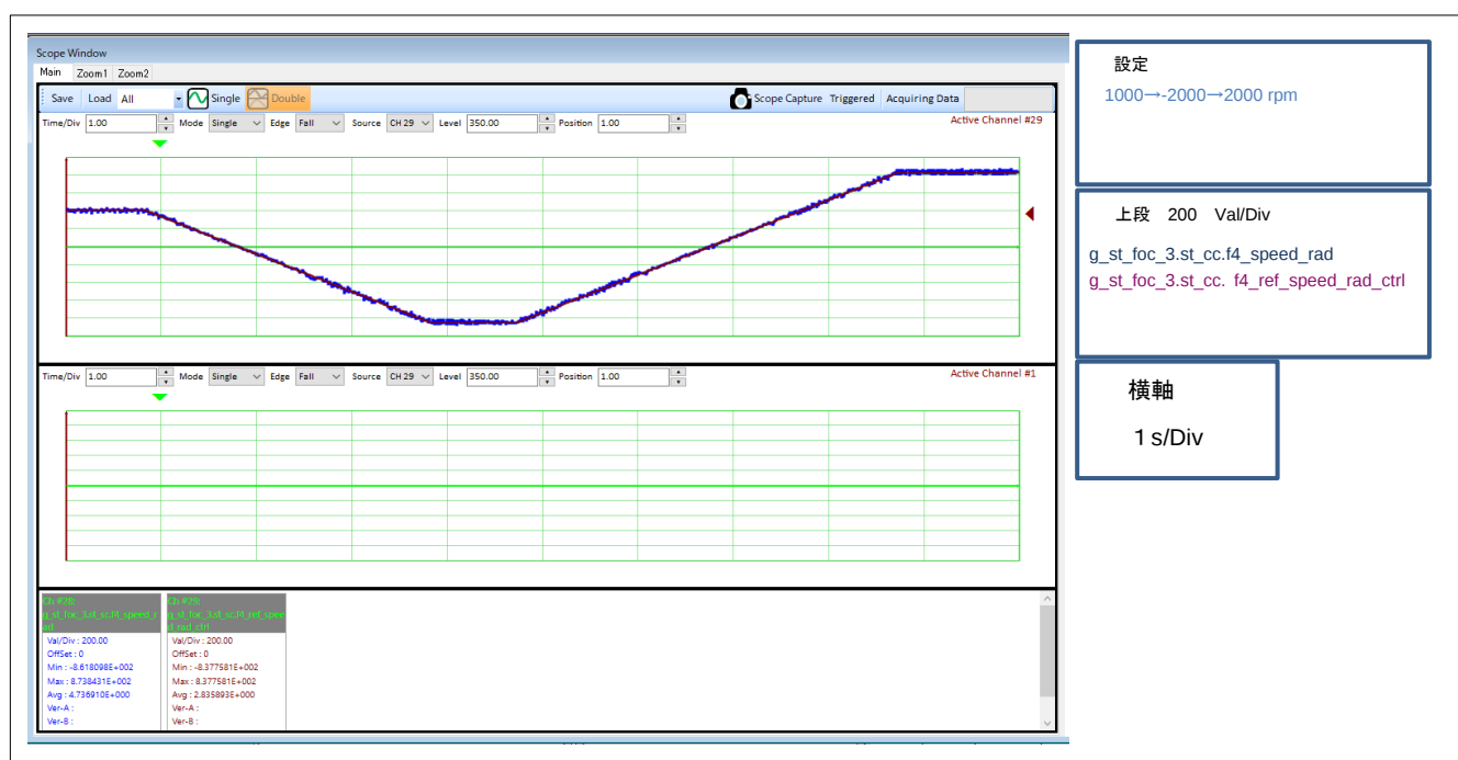
図 5-6 過渡時駆動波形（2/2）（モータ 3）
