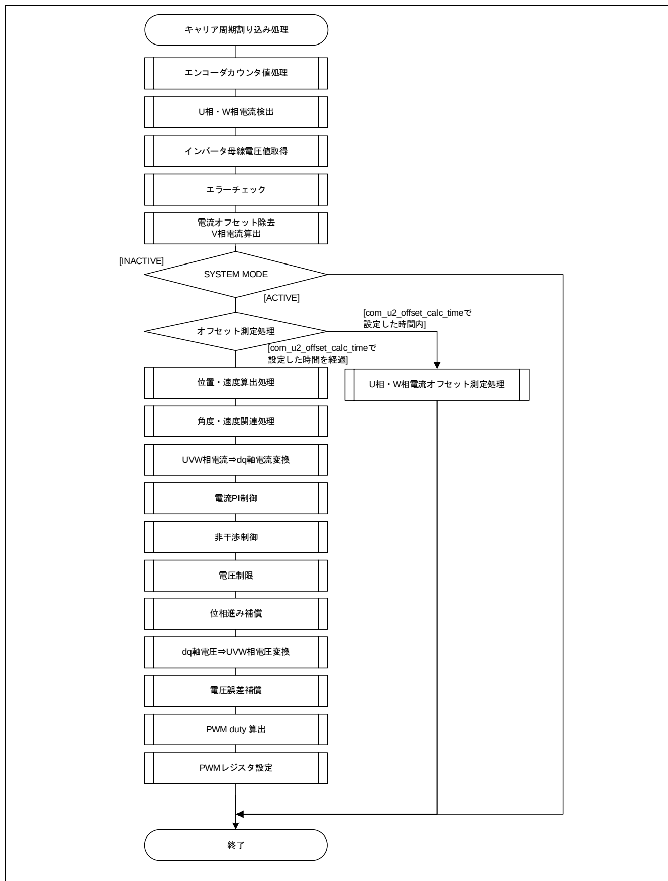
図 3-11 キャリア周期割り込み処理フローチャート（50 [μs]）
