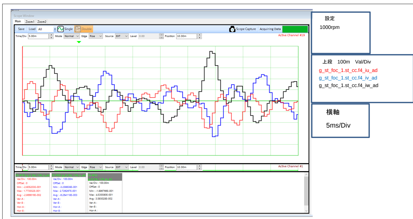
図 5-4 モータ 1 定常時駆動波形
