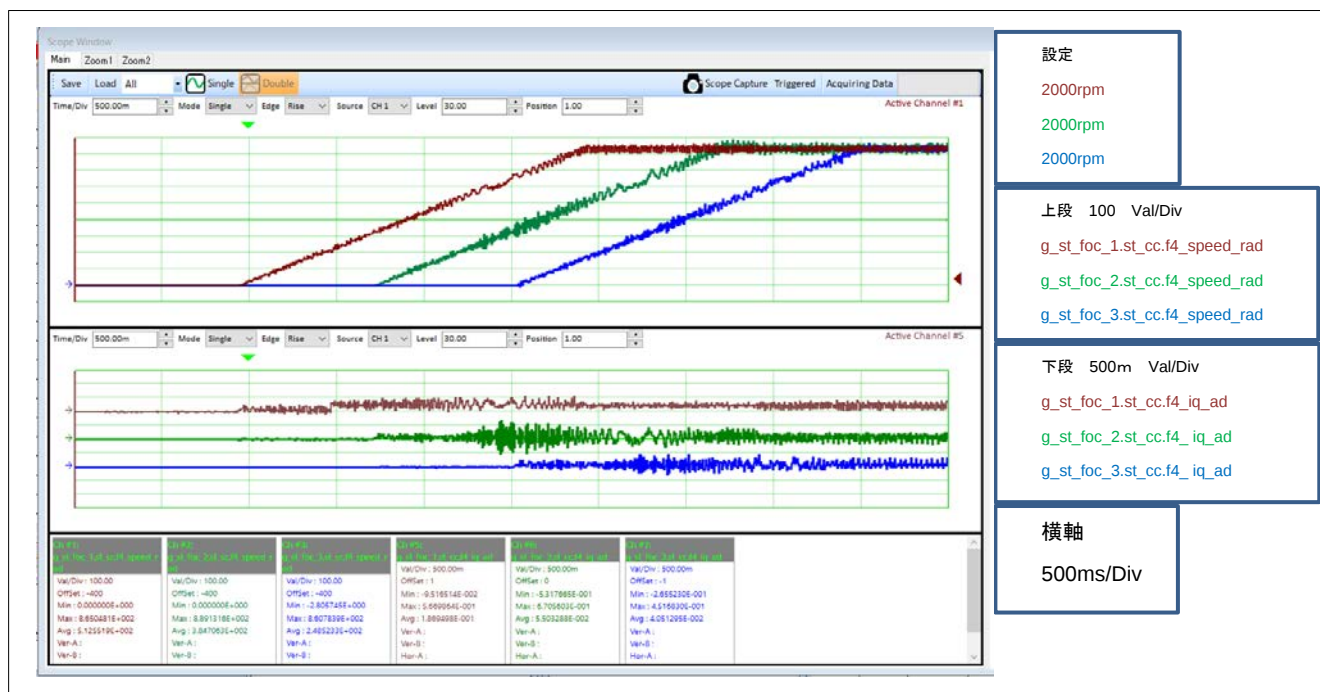
図 5-1 起動時駆動波形（1/3）（モータ 1、モータ 2、モータ 3）
