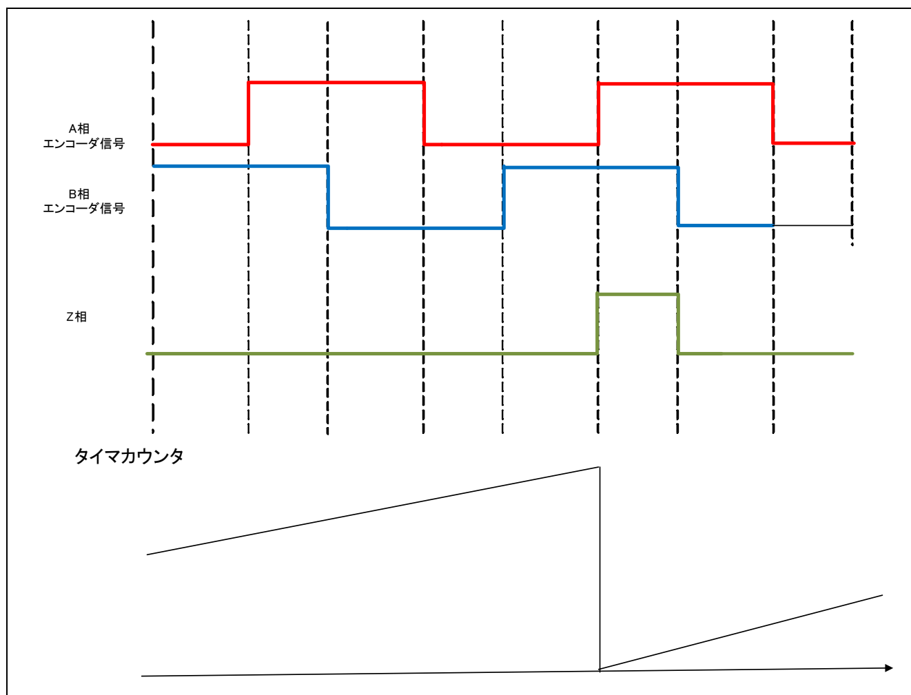
図 3-3 Z 相検出によるタイマカウンタクリア
