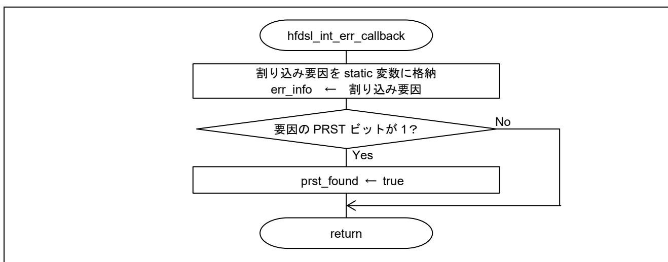
図 4-10 hfdsl_int_err_callback 関数のフローチャート
