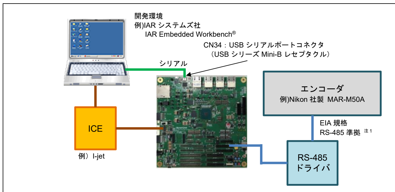
図 1-1 動作環境
