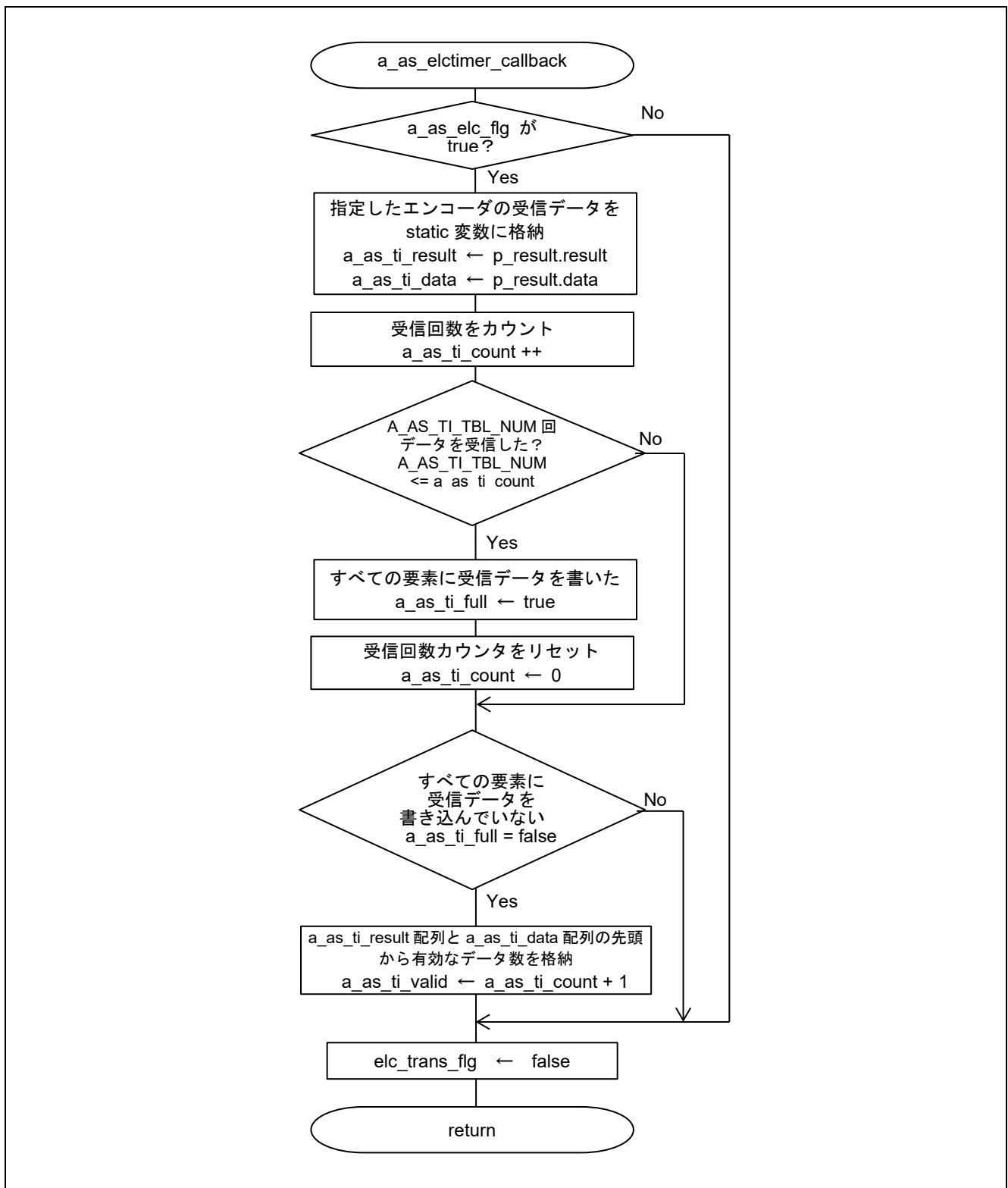
図 4-10 a_as_elctimer_callback 関数のフローチャート
