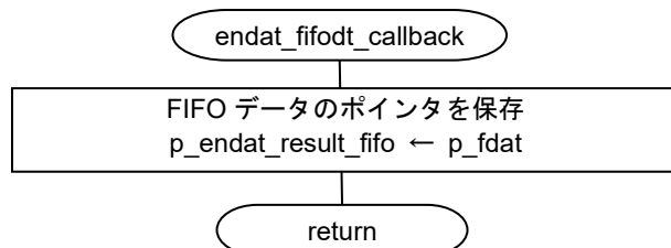
図 4-18 endat_fifodt_callback 関数のフローチャート
