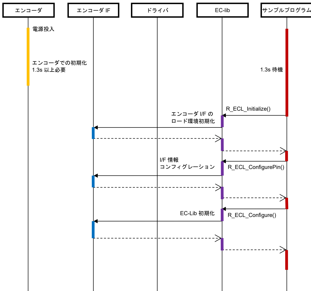
図 4-20 起動シーケンス図
