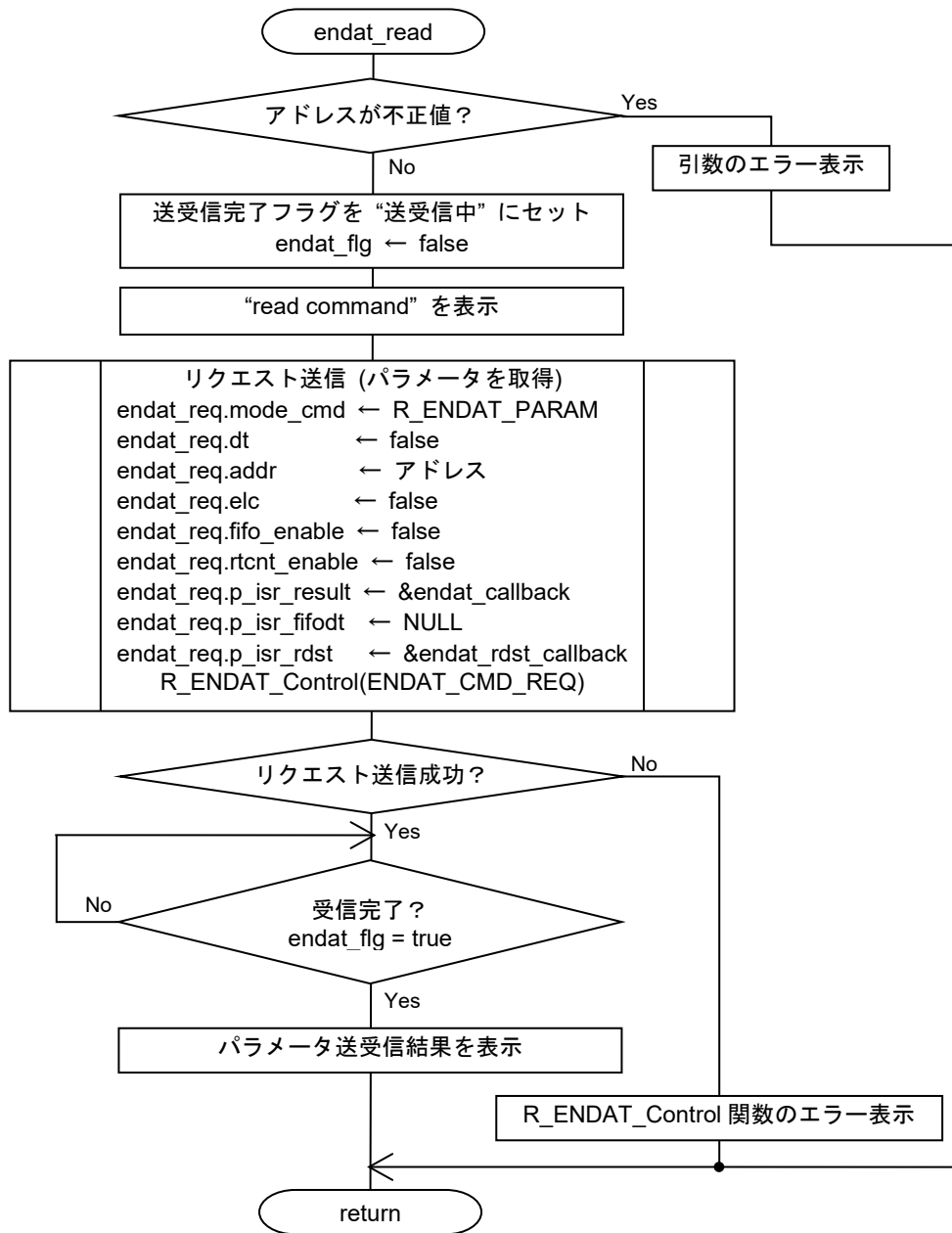
図 4-10 endat_read 関数のフローチャート
