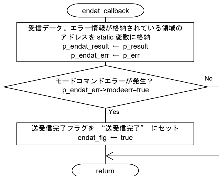
図 4-16 endat_callback 関数のフローチャート
