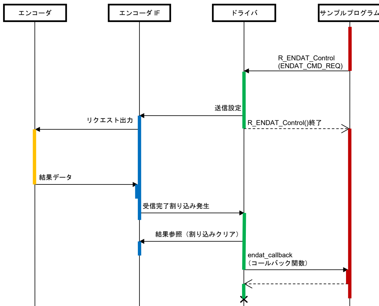
図 4-22 リクエスト送信とデータ受信のシーケンス図
