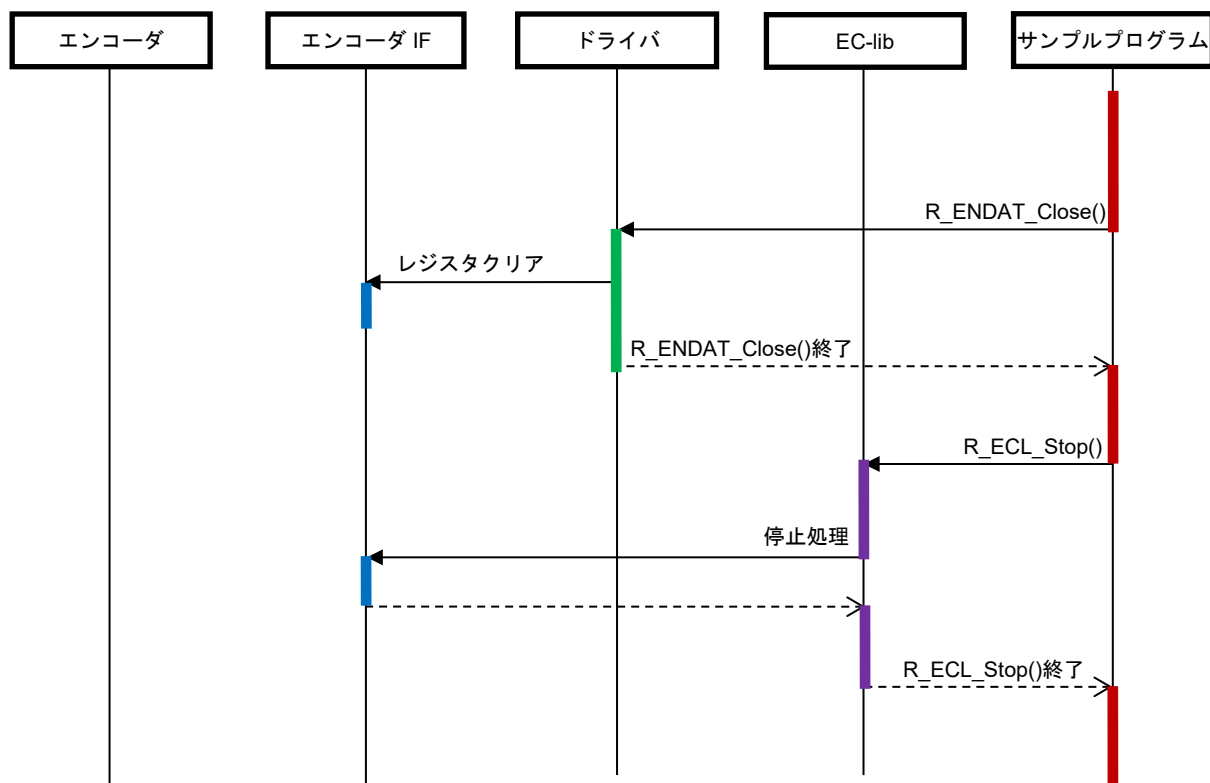
図 4-25 停止シーケンス図
