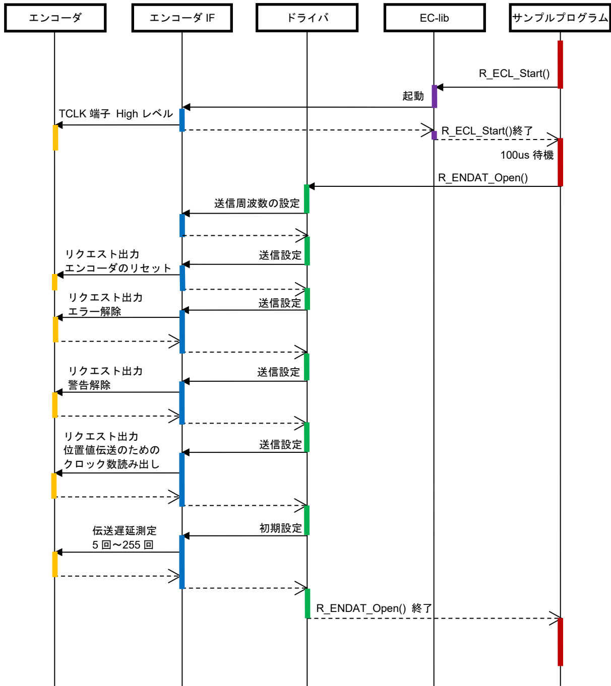
図 4-21 開始シーケンス図
