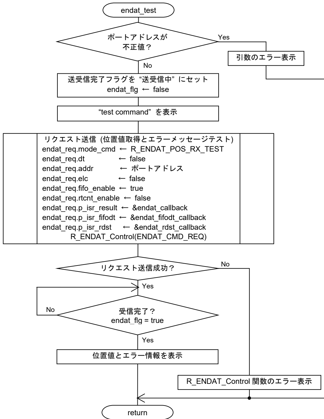
図 4-15 endat_test 関数のフローチャート
