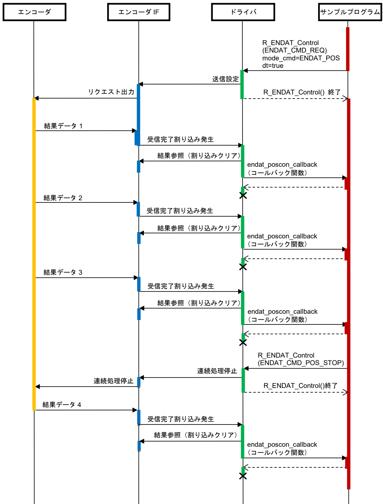
図 4-23 リクエスト送信(Continuous モード)とデータの連続受信シーケンス図
