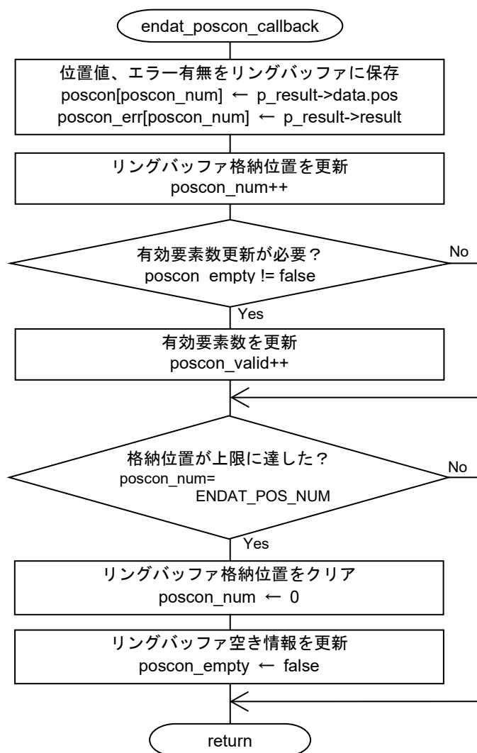
図 4-17 endat_poscon_callback 関数のフローチャート
