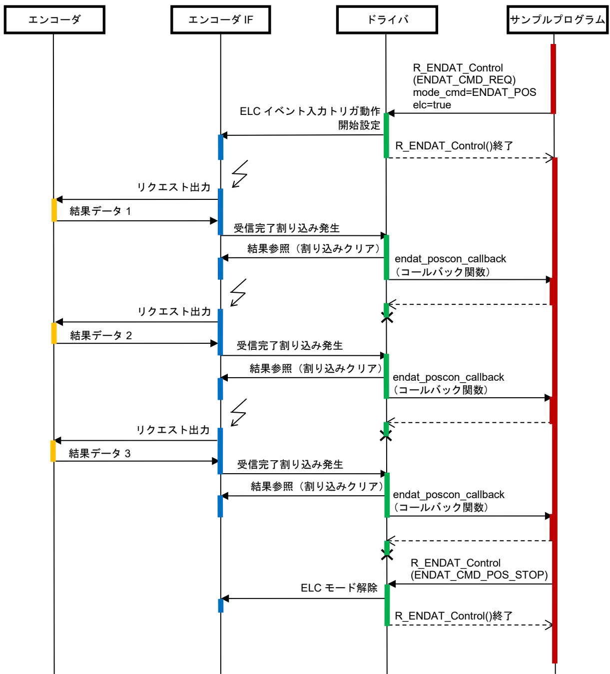
図 4-24 リクエスト送信(ELC モード)とデータの連続受信シーケンス図
