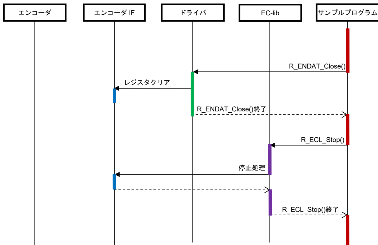
図 4-18 停止シーケンス図
