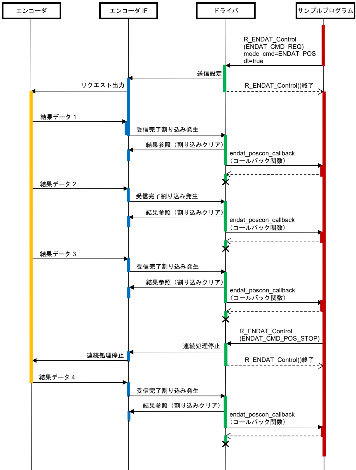
図 4-16 リクエスト送信(Continuous モード)とデータの連続受信シーケンス図
