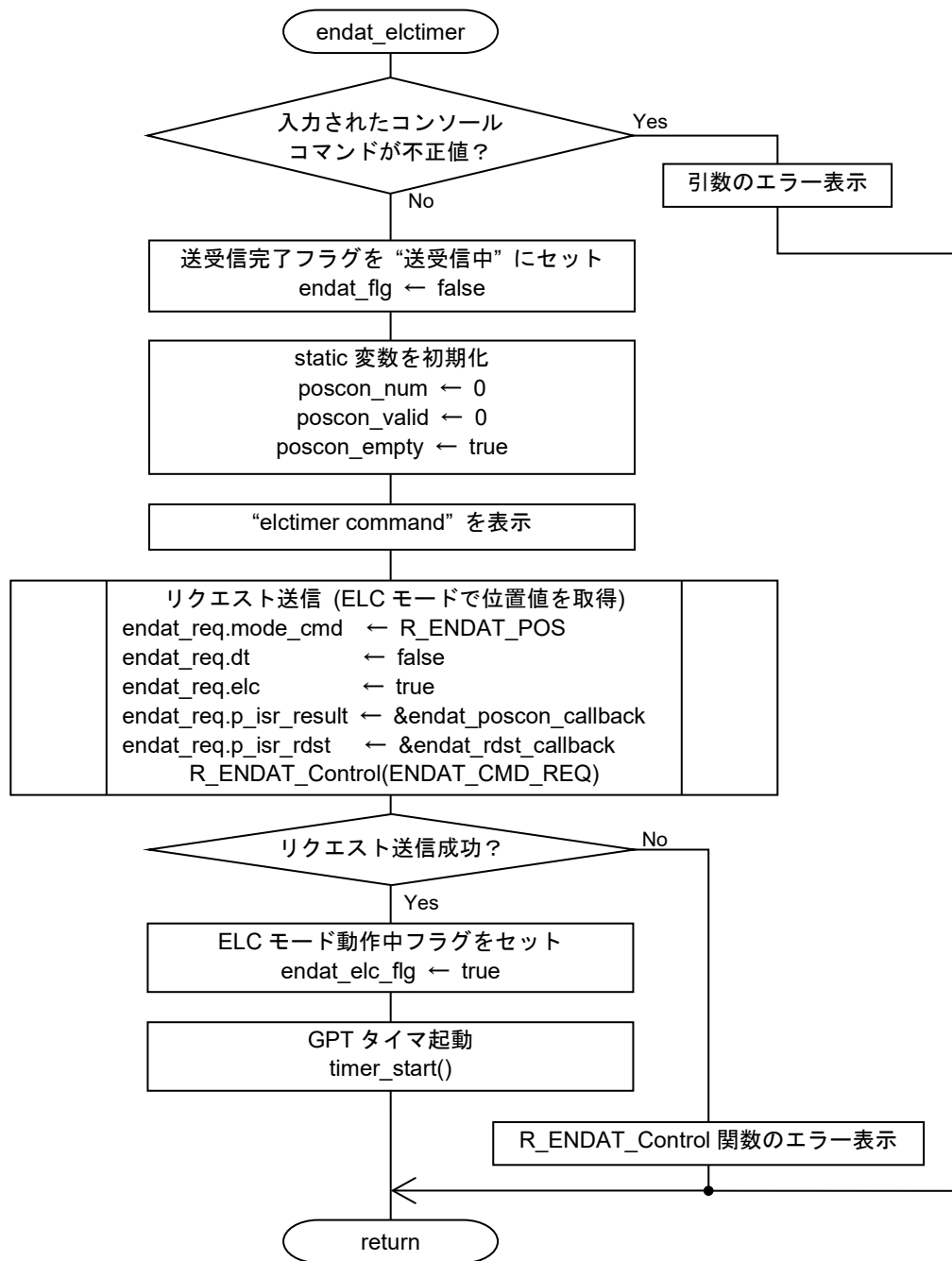
図 4-7 endat_elctimer 関数のフローチャート
