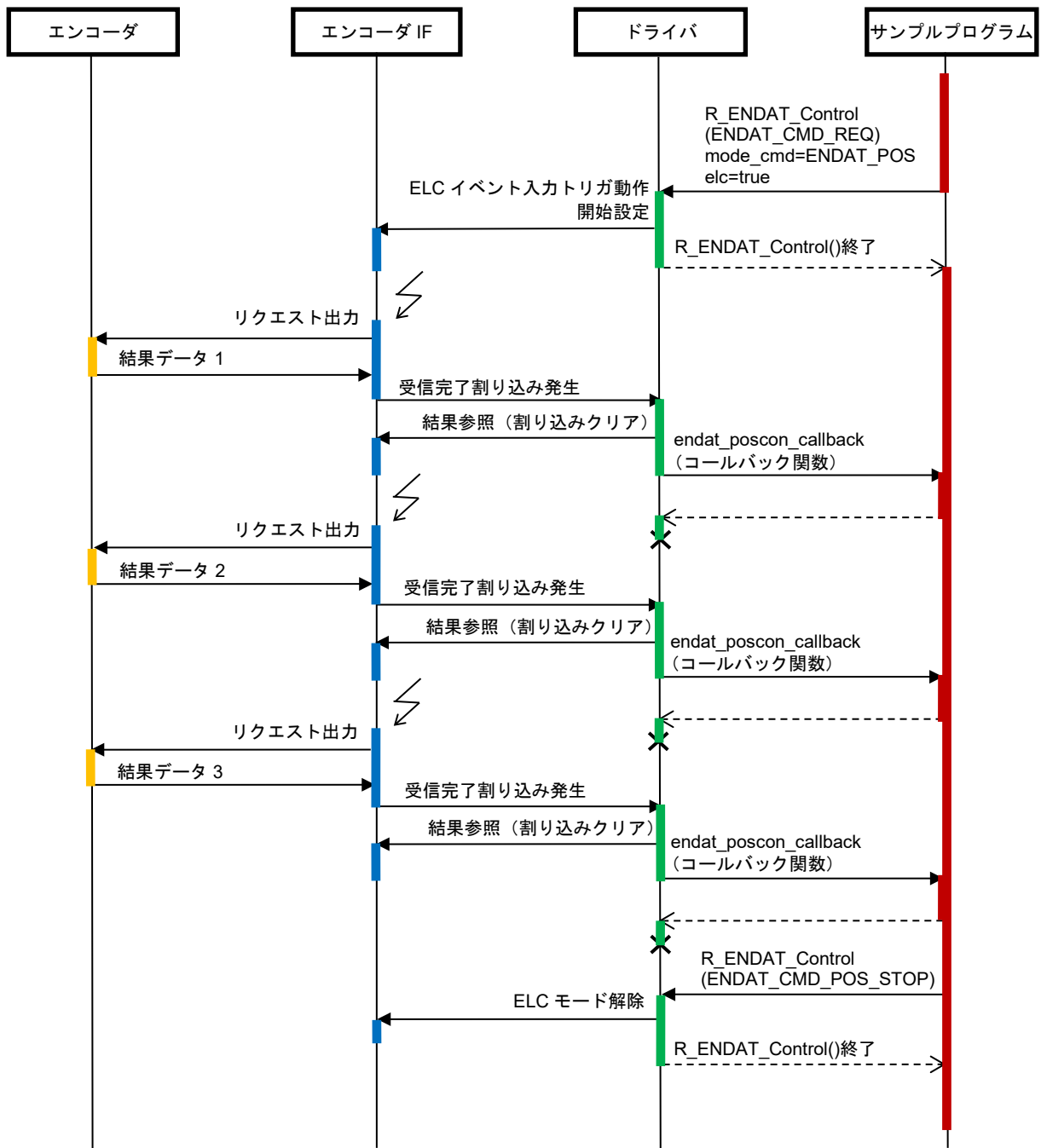
図 4-17 リクエスト送信(ELC モード)とデータの連続受信シーケンス図
