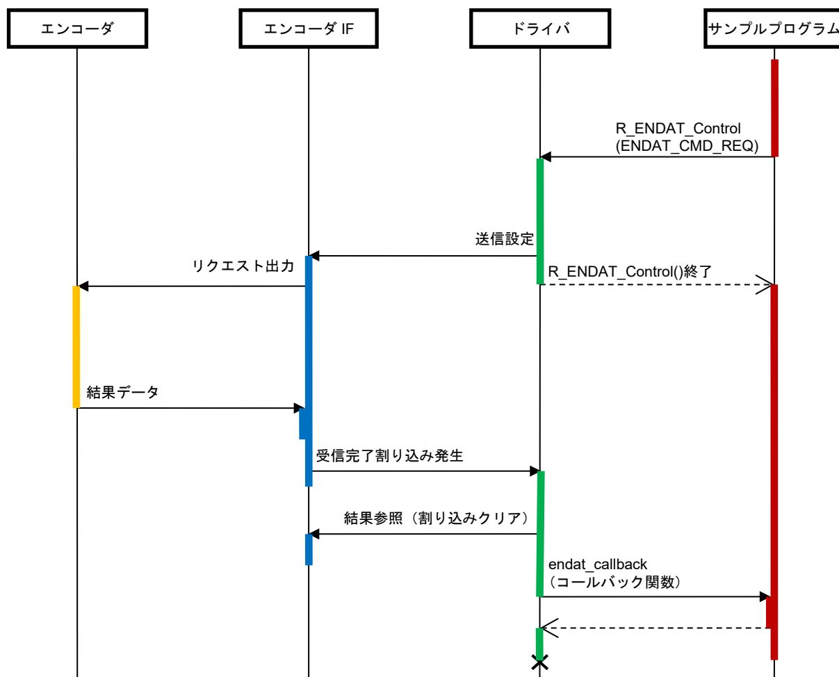
図 4-15 リクエスト送信とデータ受信のシーケンス図
