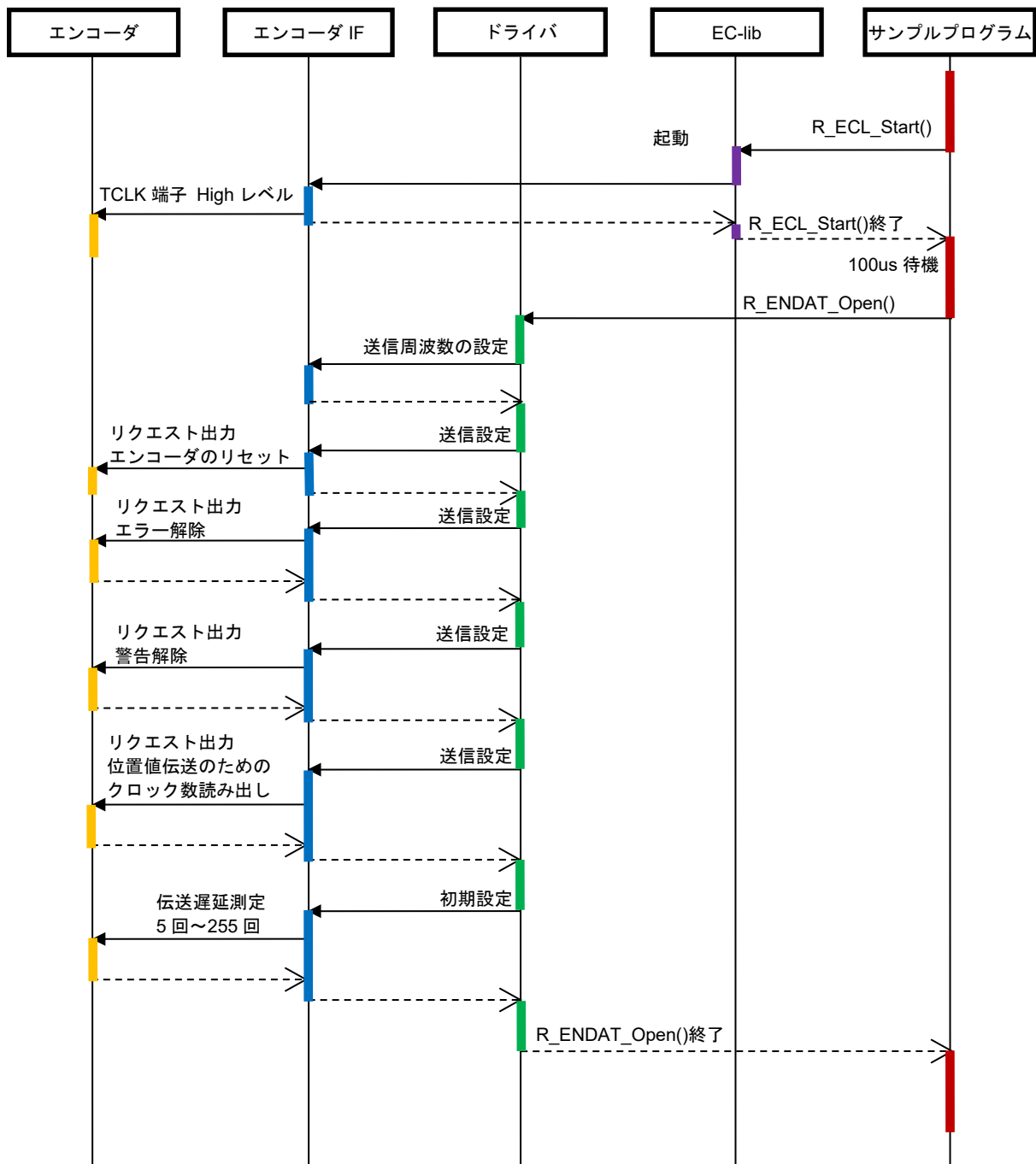
図 4-14 開始シーケンス図
