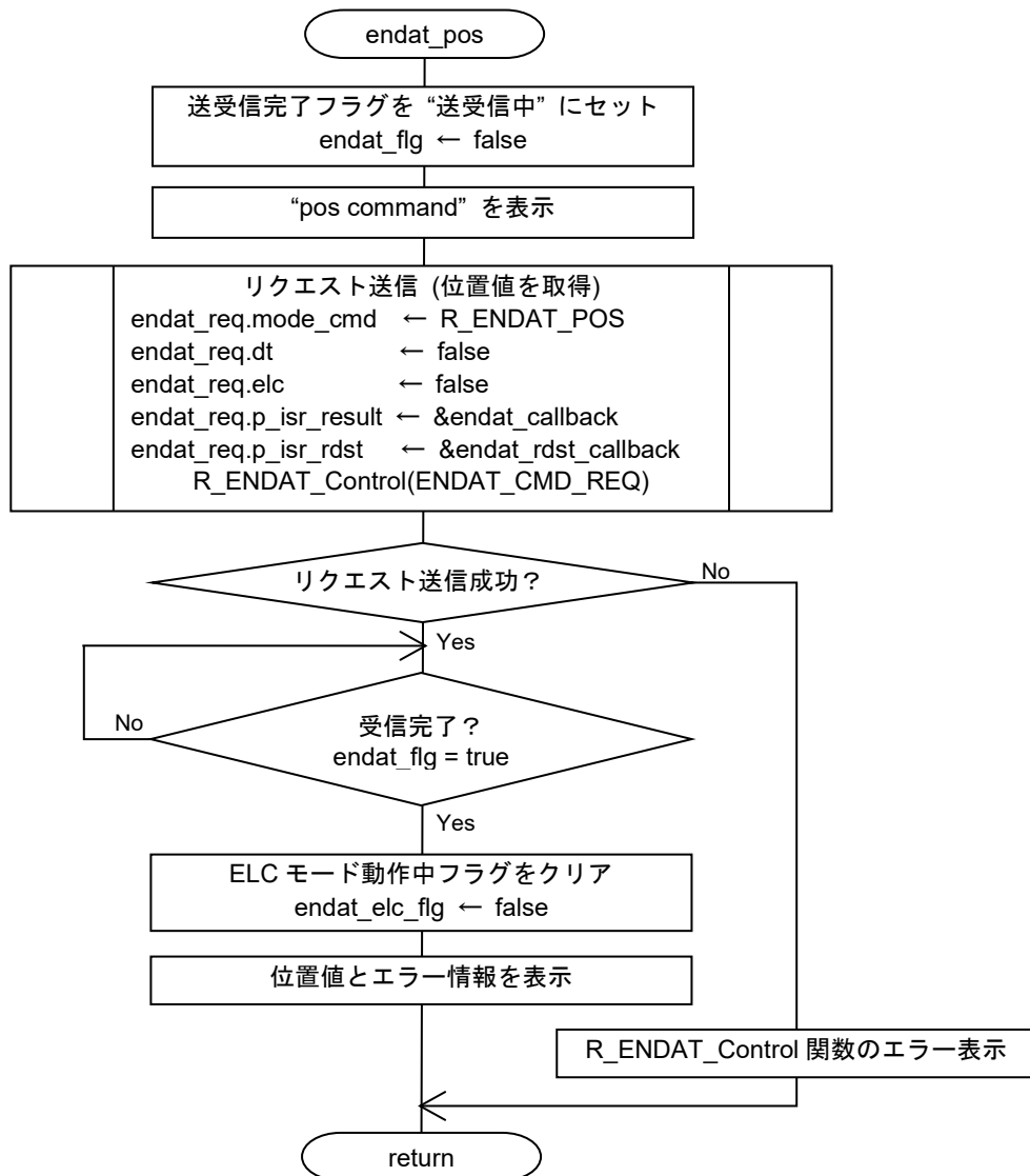
図 4-5 endat_pos 関数のフローチャート
