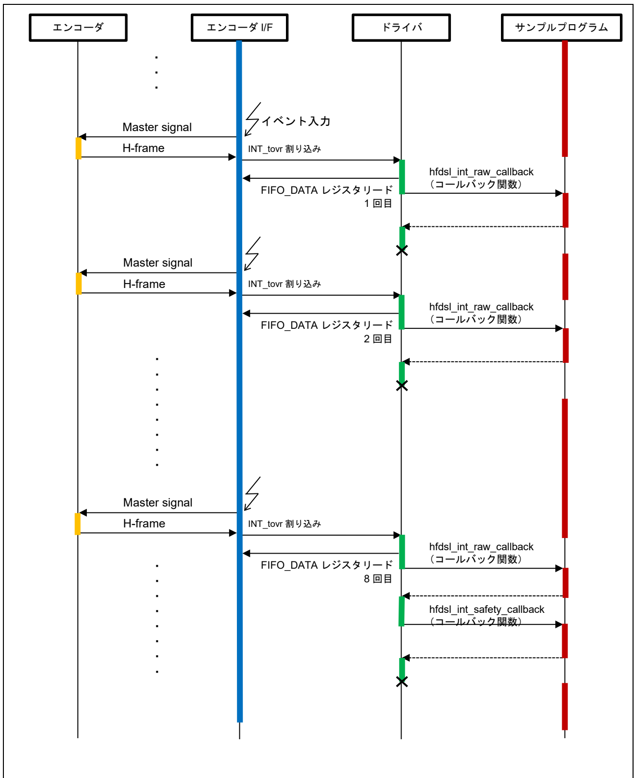
図 4-22 Vertical channel / Secondary channel データ取得シーケンス図
