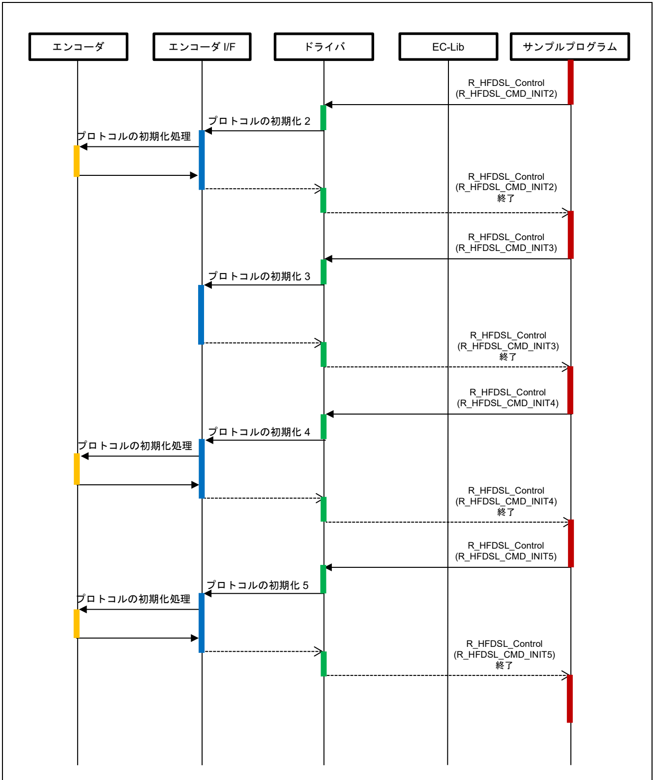
図 4-18 開始シーケンス図(2/3)
