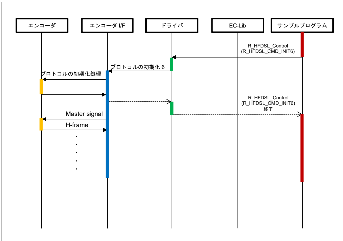
図 4-19 開始シーケンス図(3/3)
