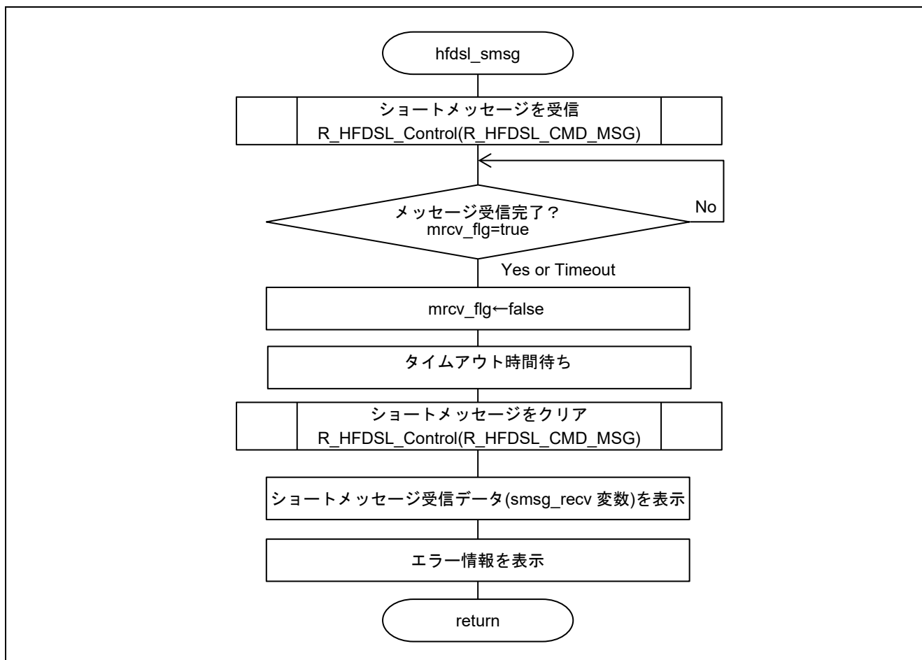
図 4-9 hfdsl_smsg 関数のフローチャート
