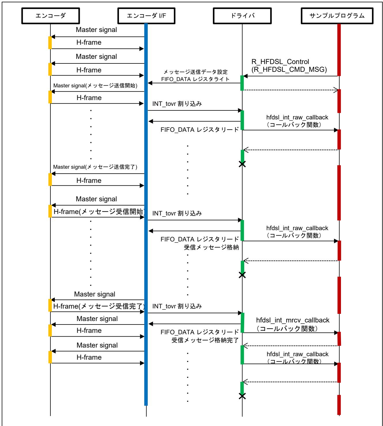
図 4-23 メッセージ送受信シーケンス図
