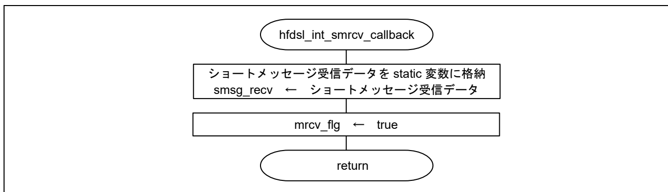
図 4-15 hfdsl_int_smrcv_callback 関数のフローチャート
