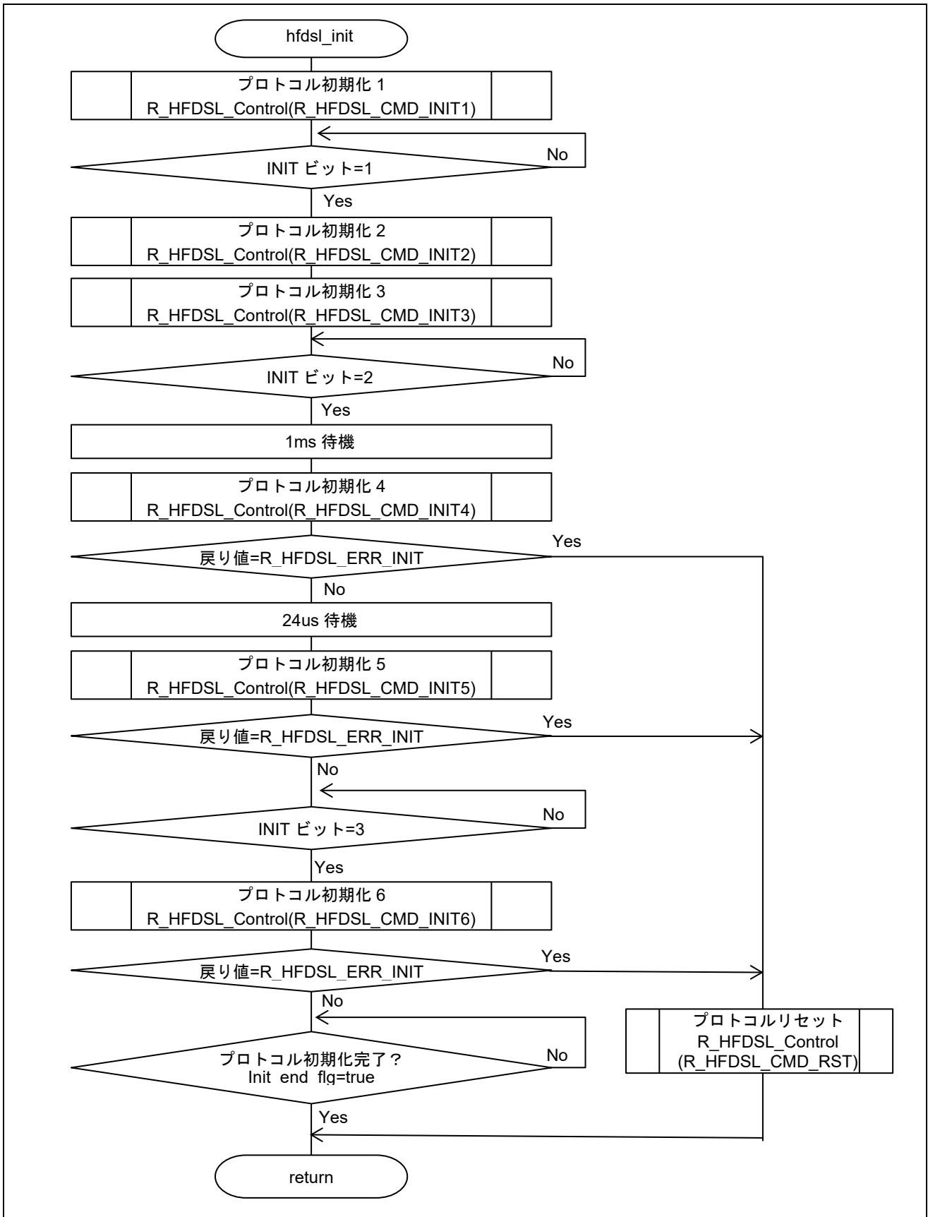
図 4-6 hfds_init 関数のフローチャート
