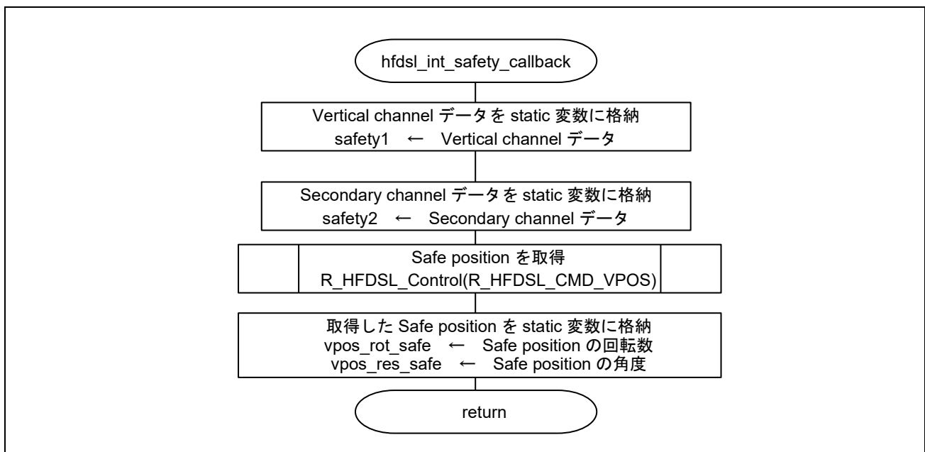
図 4-13 hfdsI_int_safety_callback 関数のフローチャート
