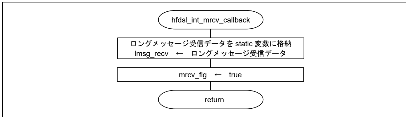
図 4-14 hfdsl_int_mrcv_callback 関数のフローチャート
