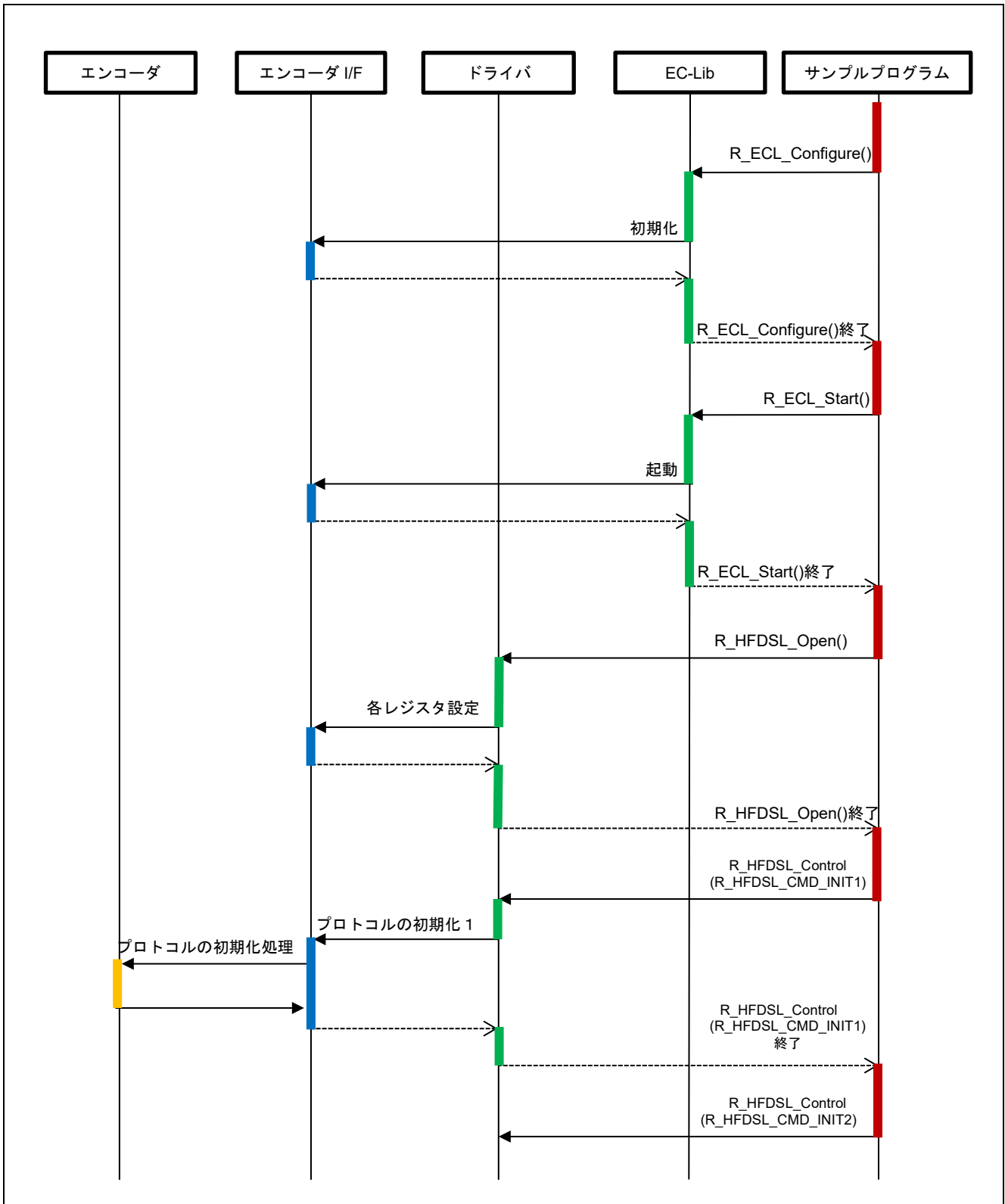
図 4-17 開始シーケンス図(1/3)
