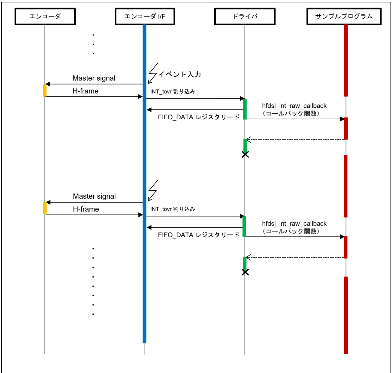
図 4-21 Sensor Hub channel データ取得シーケンス図
