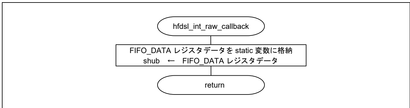
図 4-12 hfdsI_int_raw_callback 関数のフローチャート
