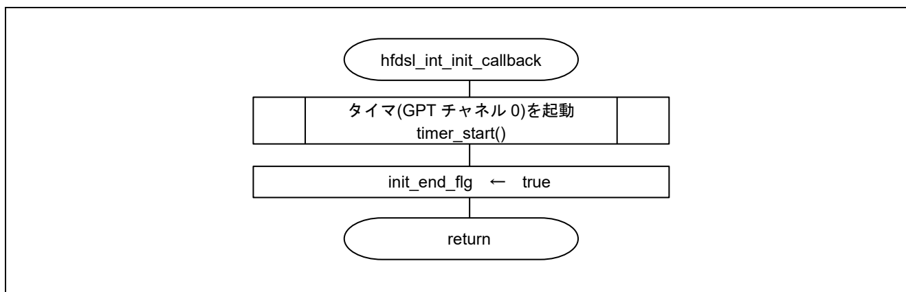
図 4-16 hfdsl_int_init_callback 関数のフローチャート
