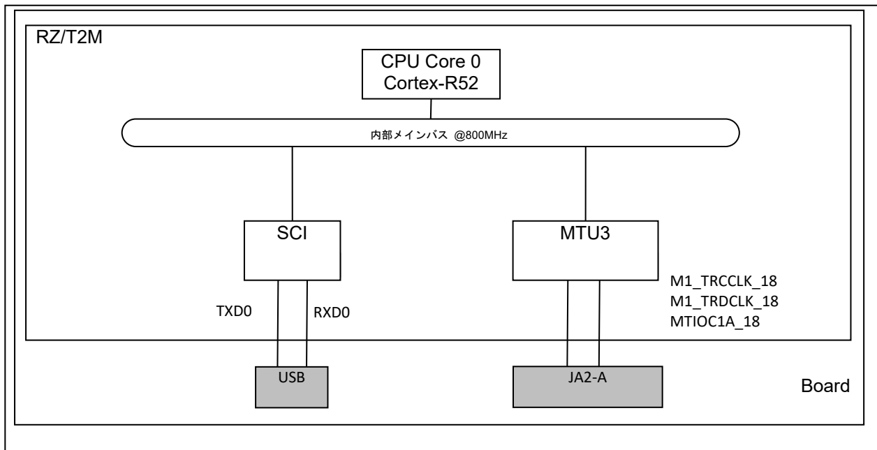
図 4.1 ハードウェア構成 (RZ/T2M)
