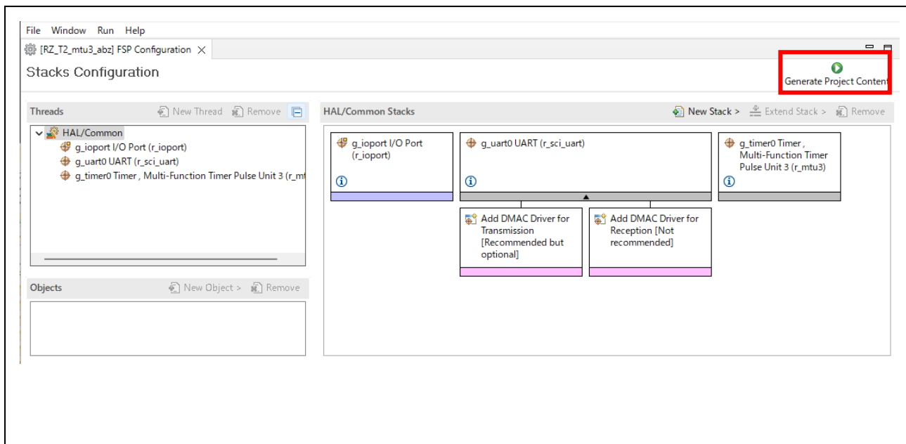
図 6.3 コード生成
