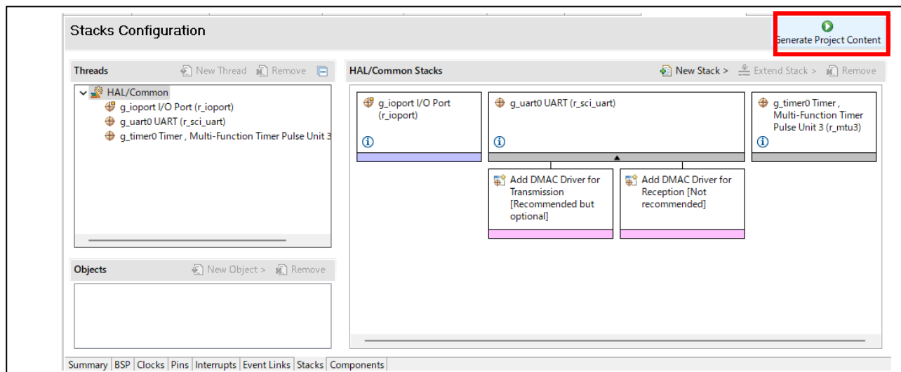
図 6.9 コード生成
