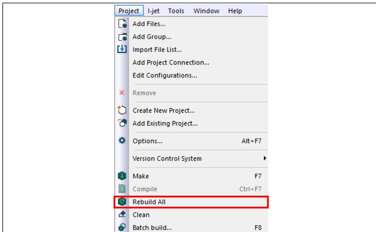
図 6.4 Rebuild All
