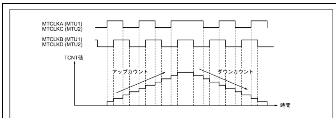
図 17.31 位相計数モード 1 の動作例
