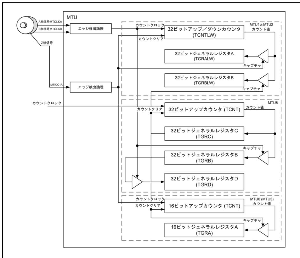
図 7.2 カスケード接続 32 ビット位相計数モード
