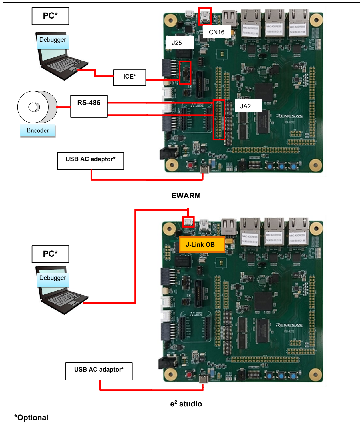
図 1.1 動作環境 (RZ/T2M)
