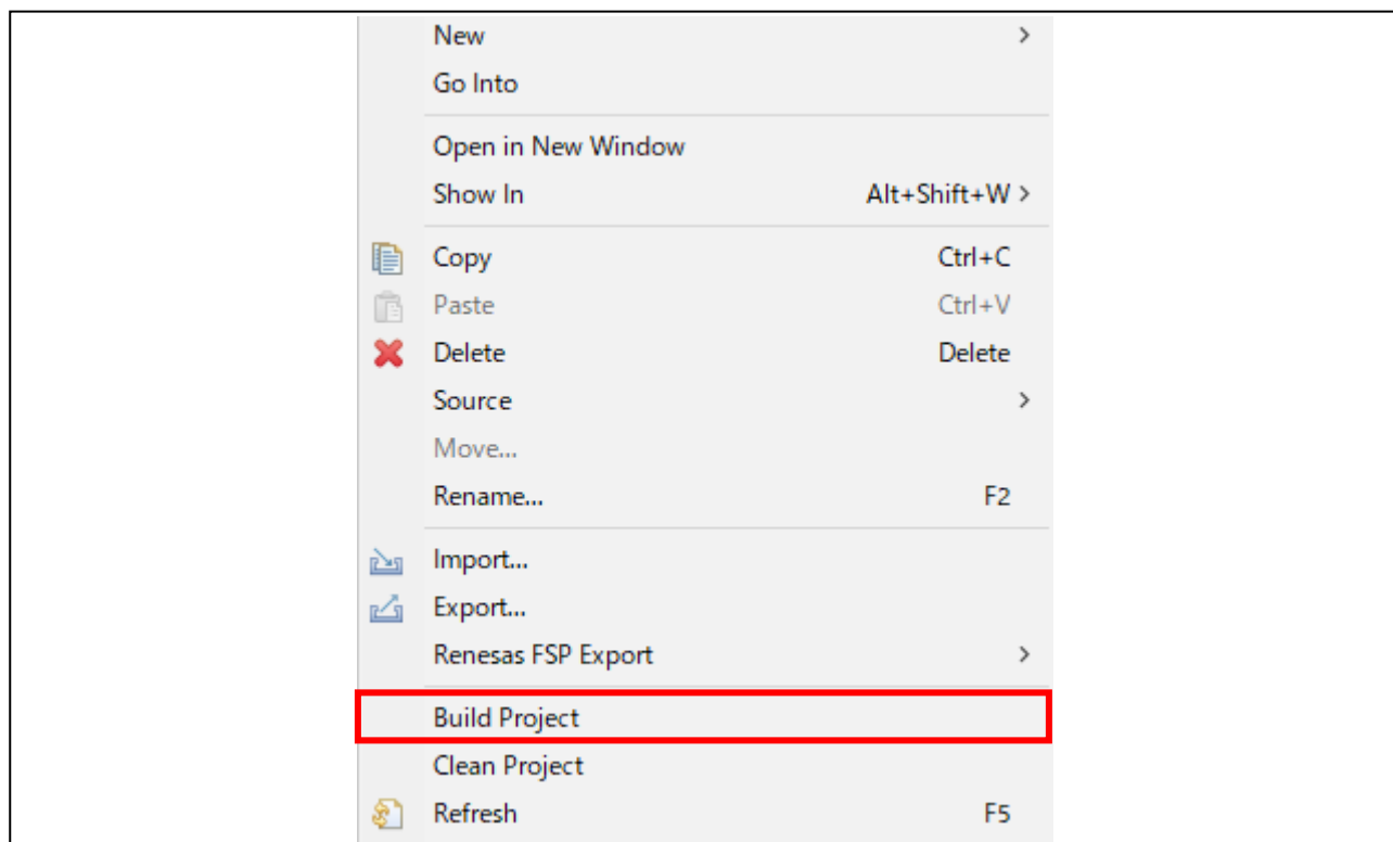
図 6.10 ビルド実行
