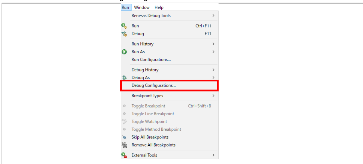
図 6.11 Debug Configurations
