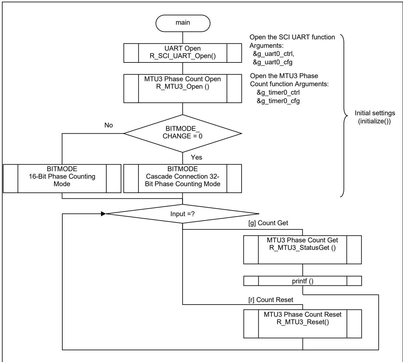
図 5.2 フローチャート (初期化、モード選択)
