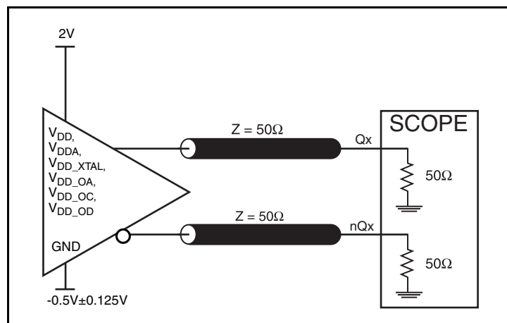
2.5V Core/2.5V LVPECL Output Load Test Circuit
