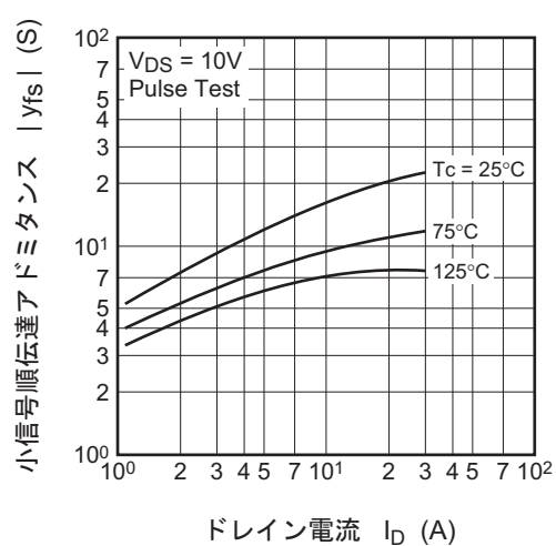
小信号順伝達アドミタンス— ドレイン電流特性 (代表例)
