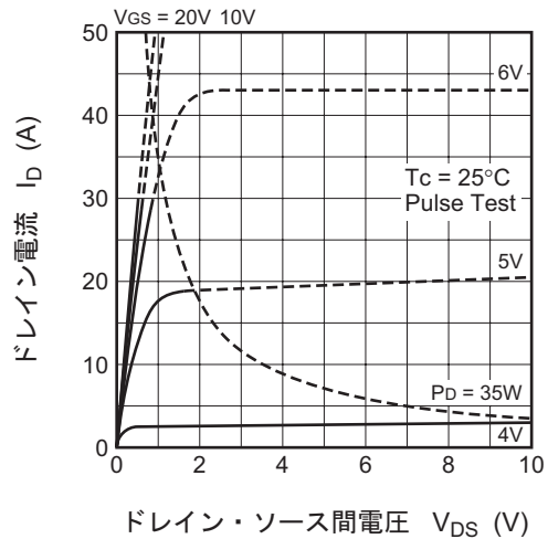
ドレイン電流—ドレイン・ソース間 電圧特性 (代表例)
