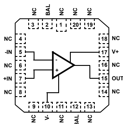
5962-896360 (CLCC)
