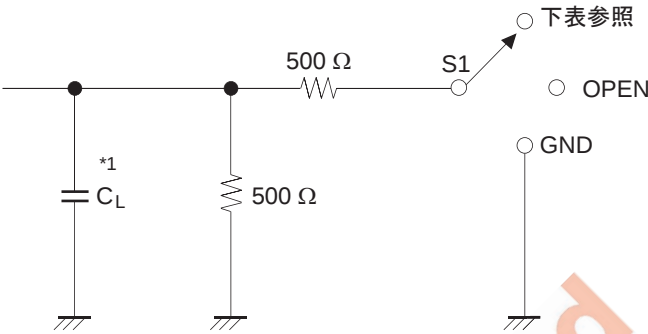
負 荷 回 路
