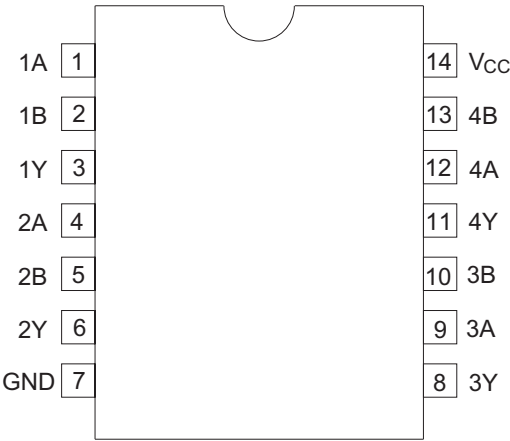
(上面図)
