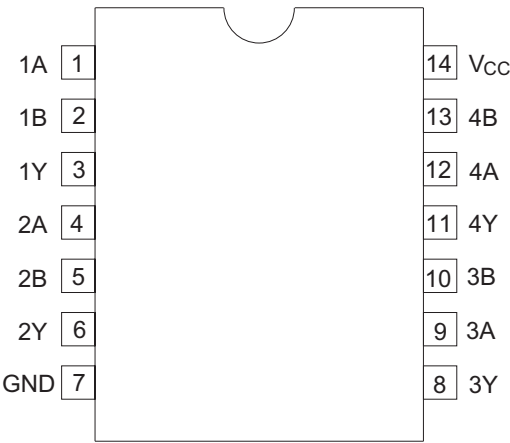
(上面図)
