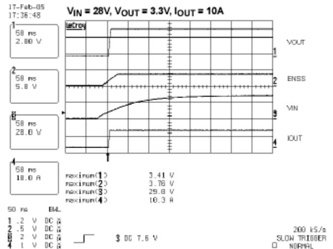
图 9 典型的软启动波形
