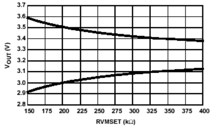
图 10 电压余量和 VMSET 电阻器数值的关系
