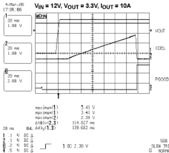
图 11 PGOOD 信号的延时
