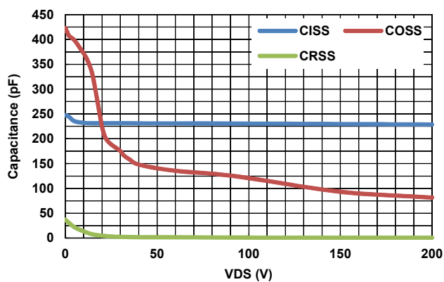
Figure 10. Capacitance (Linear Scale)
