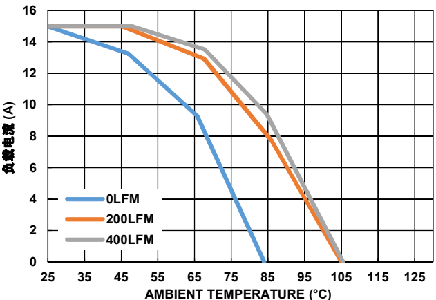
图 37. PWM/CCM 模式, V_{OUT} = 12V , f_{SW} = 600kHz
