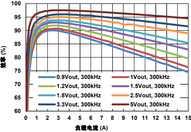
图 8。 V_{IN} = 7V
