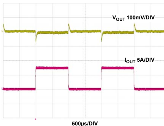
图 25。 V_{OUT} = 12\text{V} , f_{SW} = 600\text{kHz} , C_{OUT} = 12 \times 22\mu\text{F} 陶瓷 + 2 \times 150\mu\text{F} POSCAP
