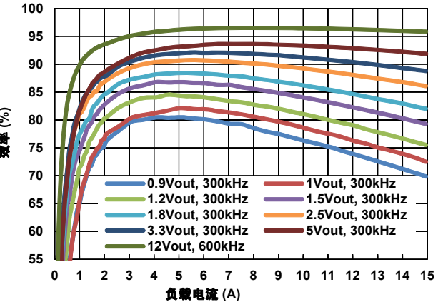
图 10。 V_{IN} = 24V
