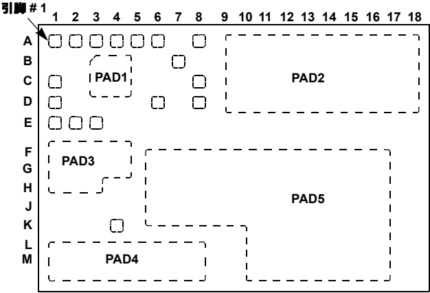
ISL8215M (22 Ld 19x13 HDA) 俯视图
