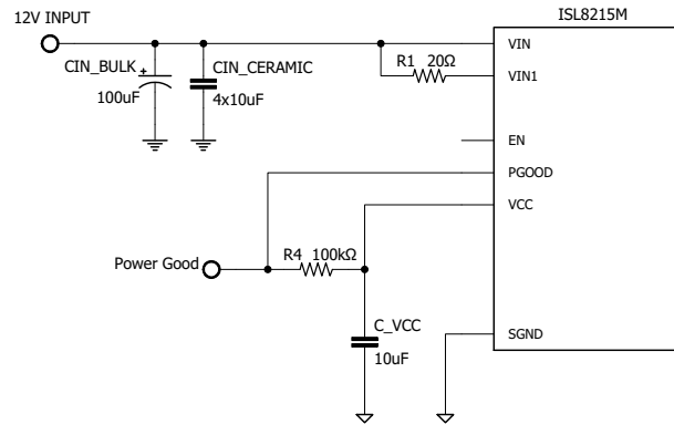
图 38。自启用操作
