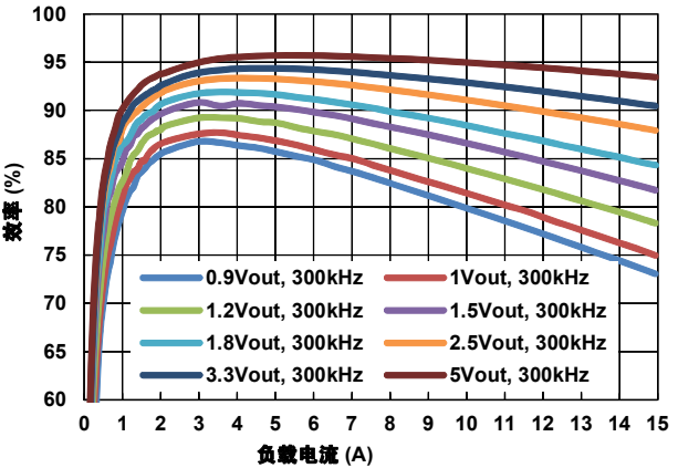
图 9。 V_{IN} = 12V
