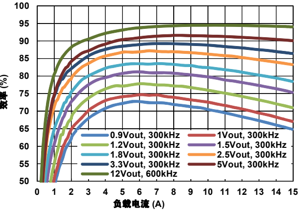
图 13。 V_{IN} = 42V
