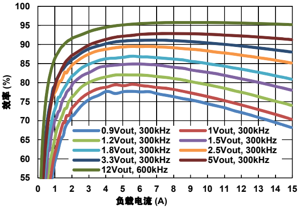
图 11。 V_{IN} = 30V
