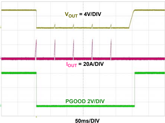
图 30。OCP 反应; 短路输出从无负载到地面, 然后释放, V_{OUT} = 5\text{V} , I_{OUT} = 0\text{A}
