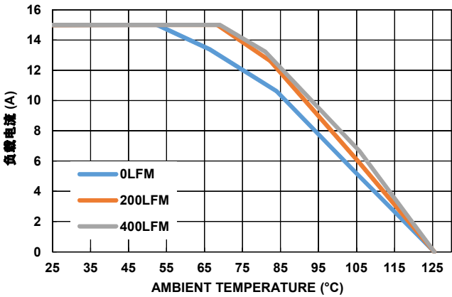
图 34. PWM/CCM 模式, V_{OUT} = 2.5V , f_{SW} = 300kHz
