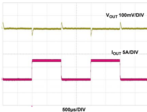
图 21。 V_{OUT} = 1.8\text{V} , f_{SW} = 300\text{kHz} , C_{OUT} = 4 \times 100\mu\text{F} 陶瓷 + 1 \times 470\mu\text{F} POSCAP
