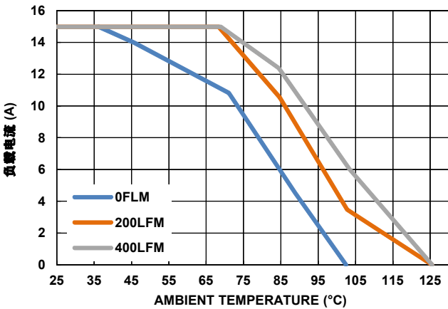
图 36. PWM/CCM 模式, V_{OUT} = 5V , f_{SW} = 300kHz
