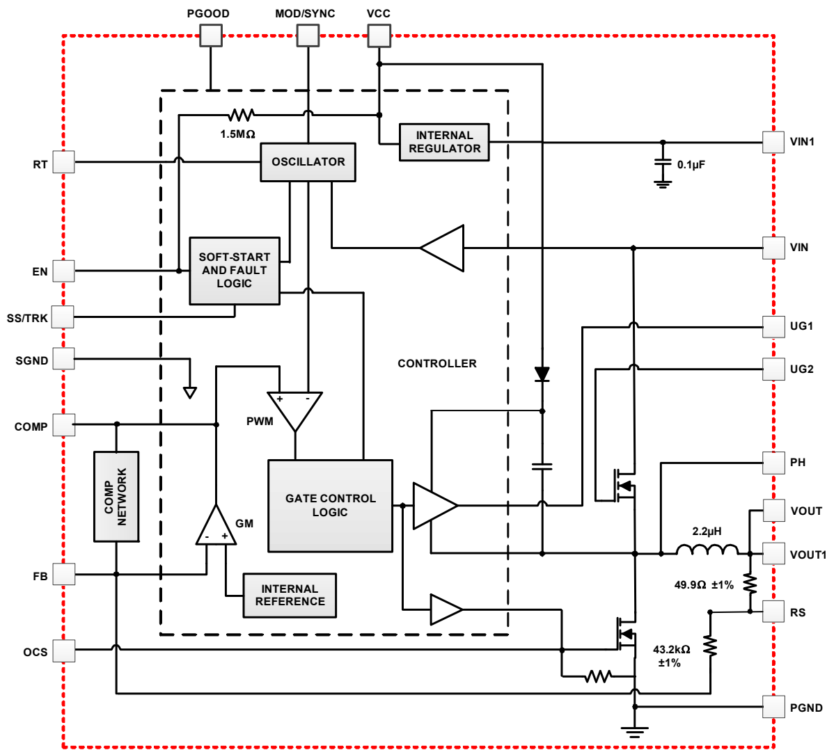
图 7。方框图
