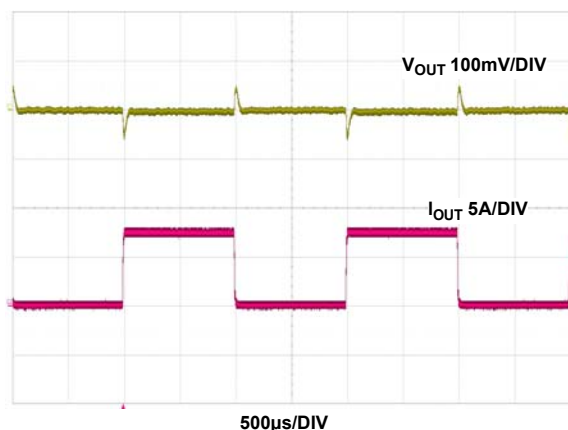
图 22。 V_{OUT} = 2.5\text{V} , f_{SW} = 300\text{kHz} , C_{OUT} = 4 \times 100\mu\text{F} 陶瓷 + 1 \times 470\mu\text{F} POSCAP
