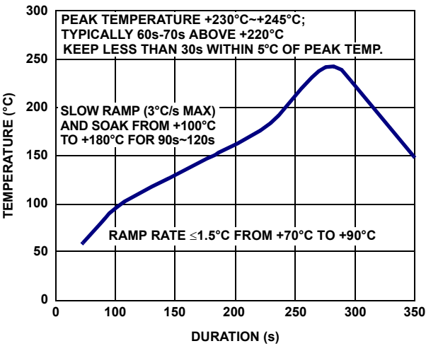
图 41. 典型回流焊曲线
