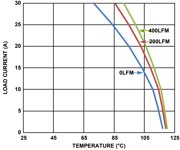
图 35. 降额曲线 5V_{IN} - 1V_{OUT}
