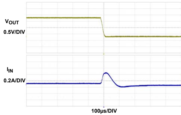
图 16. 短路 @ 0A
