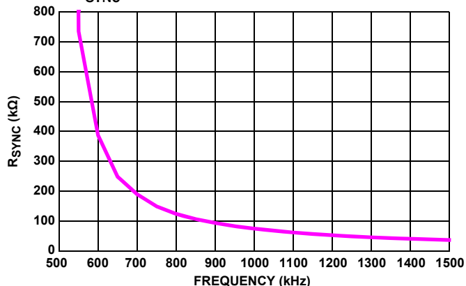
图 31. R_{SYNC} - 开关频率
