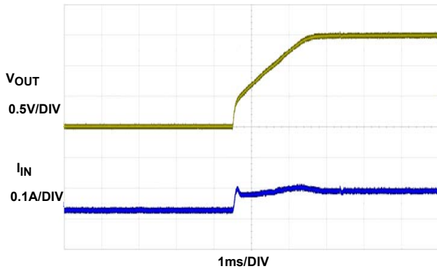
图 14. 启动 @ 0A
