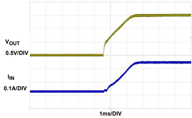
图 15. 启动 @ 15A
