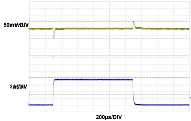
图 9.1.2 V_{OUT} 瞬态响应
