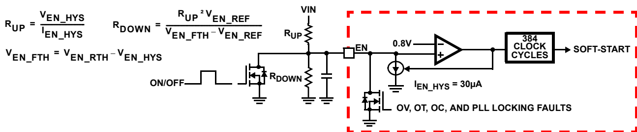
图 26. 简化的启用与电压前馈电路
