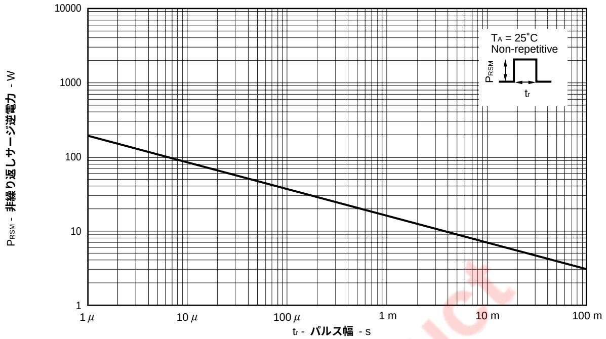
図4 サージ逆電力定格
