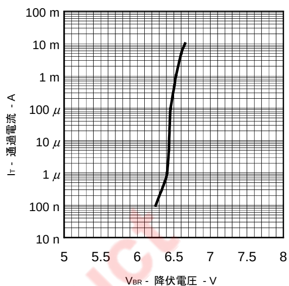
図2 I_T vs. V_{BR} 特性例
