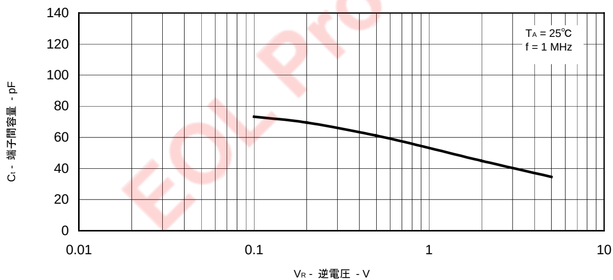
図3 C_i vs. V_R 特性例
