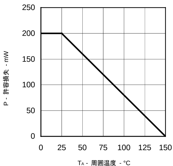
図1 P vs. T_A 定格
