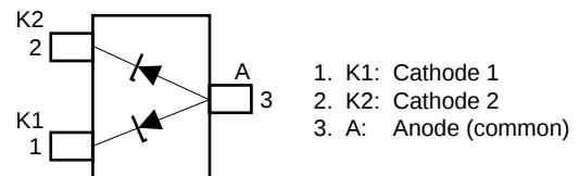
端子接続図
