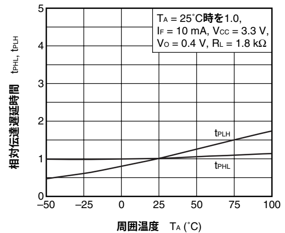
相対伝達遅延時間 vs. 周囲温度
