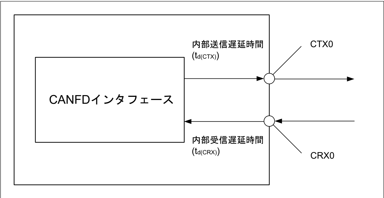
図 2.59 CANFD インタフェース条件
