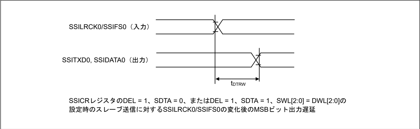
図 2.58 SSILRCK0/SSIFS0 変化時からの SSIE データ出力遅延
