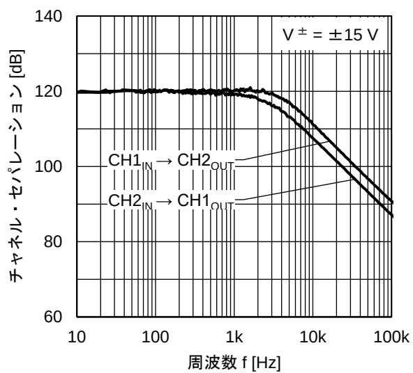
チャネル・セパレーション - f 特性
