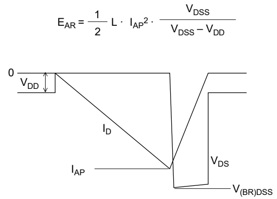
アバランシェ動作波形
