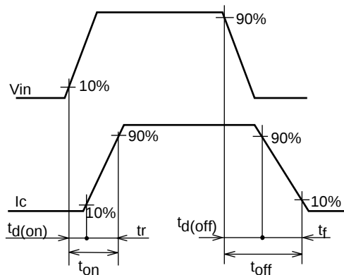
运行波形
