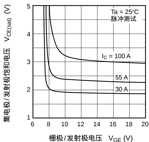
集电极/发射极饱和电压 - 栅极/发射极电压
