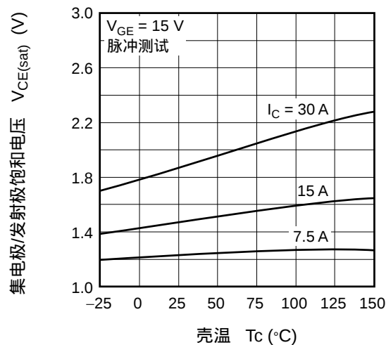
集电极/发射极饱和电压-壳温 (典型)
