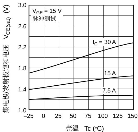
集电极/发射极饱和电压-亮温 (典型)
