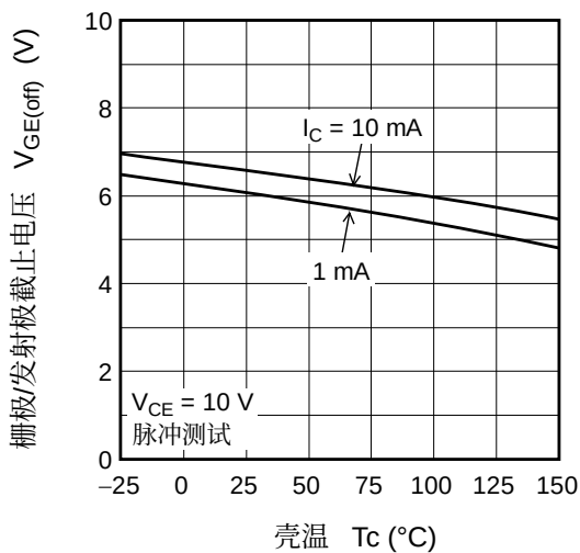
栅极/发射极截止电压-亮温 (典型)
