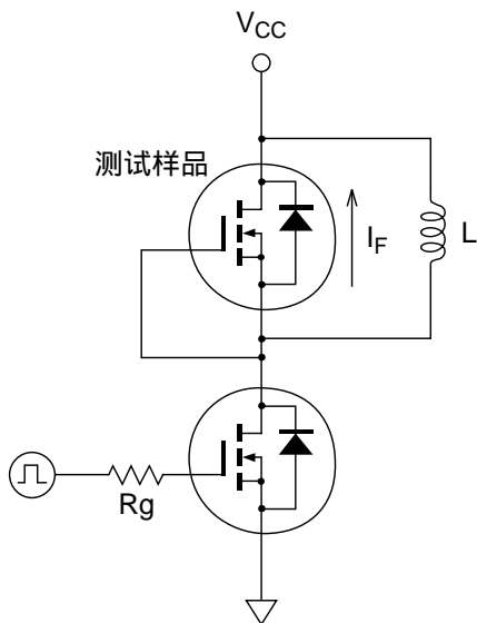
二极管反向恢复时间测定电路
