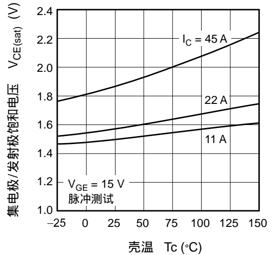
集电极/发射极饱和电压-壳温 (典型)
