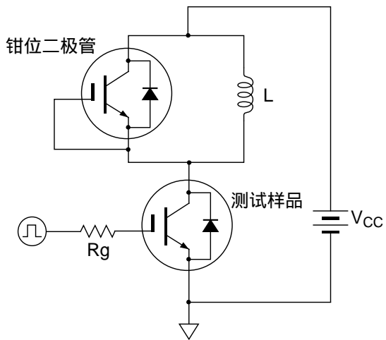
开关时间测定电路
