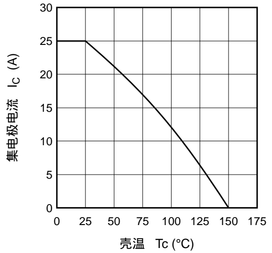
集电极最大直流电流-壳温
