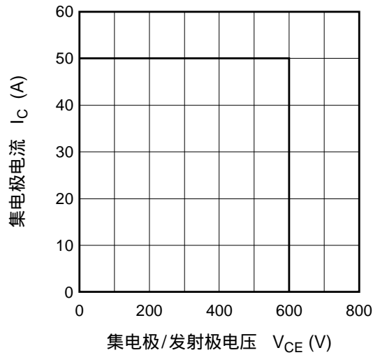
关断安全工作区域
