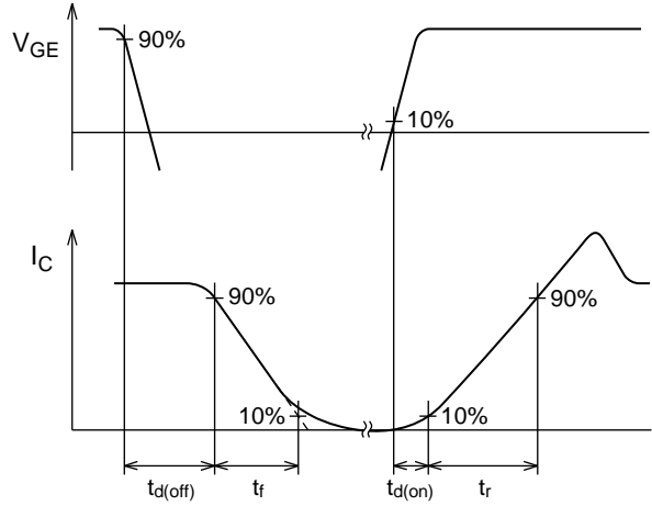
波形
