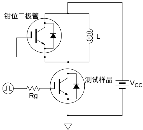
开关时间测定电路
