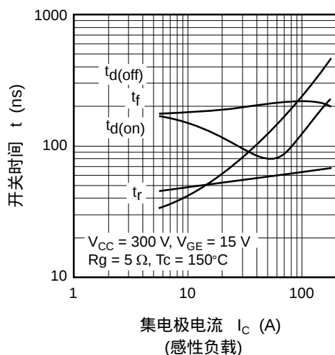
开关特性 (典型) (1)
