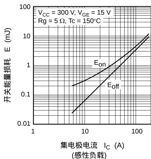
开关特性 (典型) (2)
