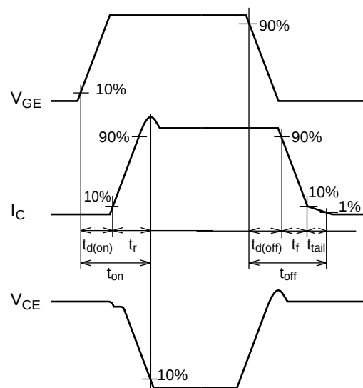
运行波形
