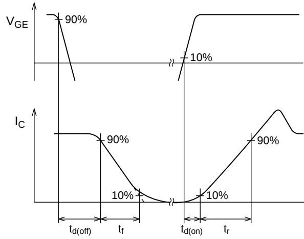
波形
